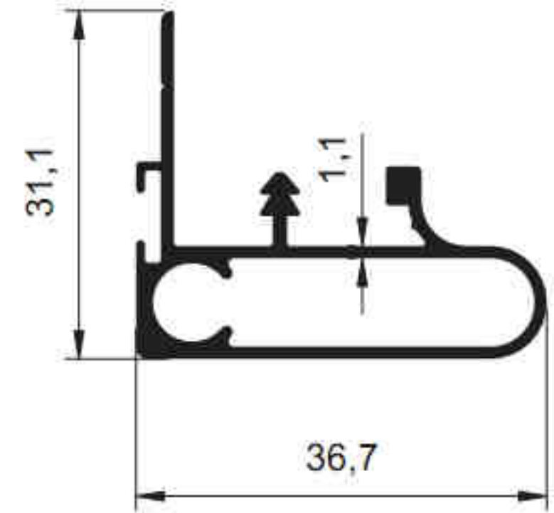
4818 - 0.457 kg/m
