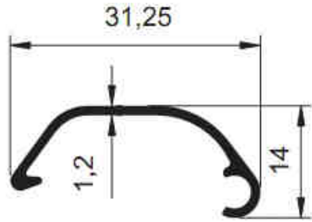
4316 - 0.490 kg/m
