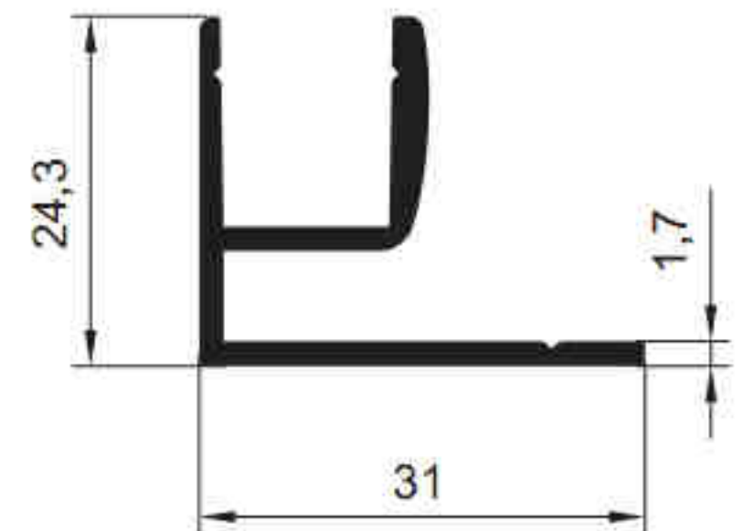
5449 - 0.389 kg/m
