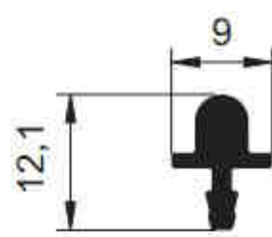
3951 - 0.128 kg/m
