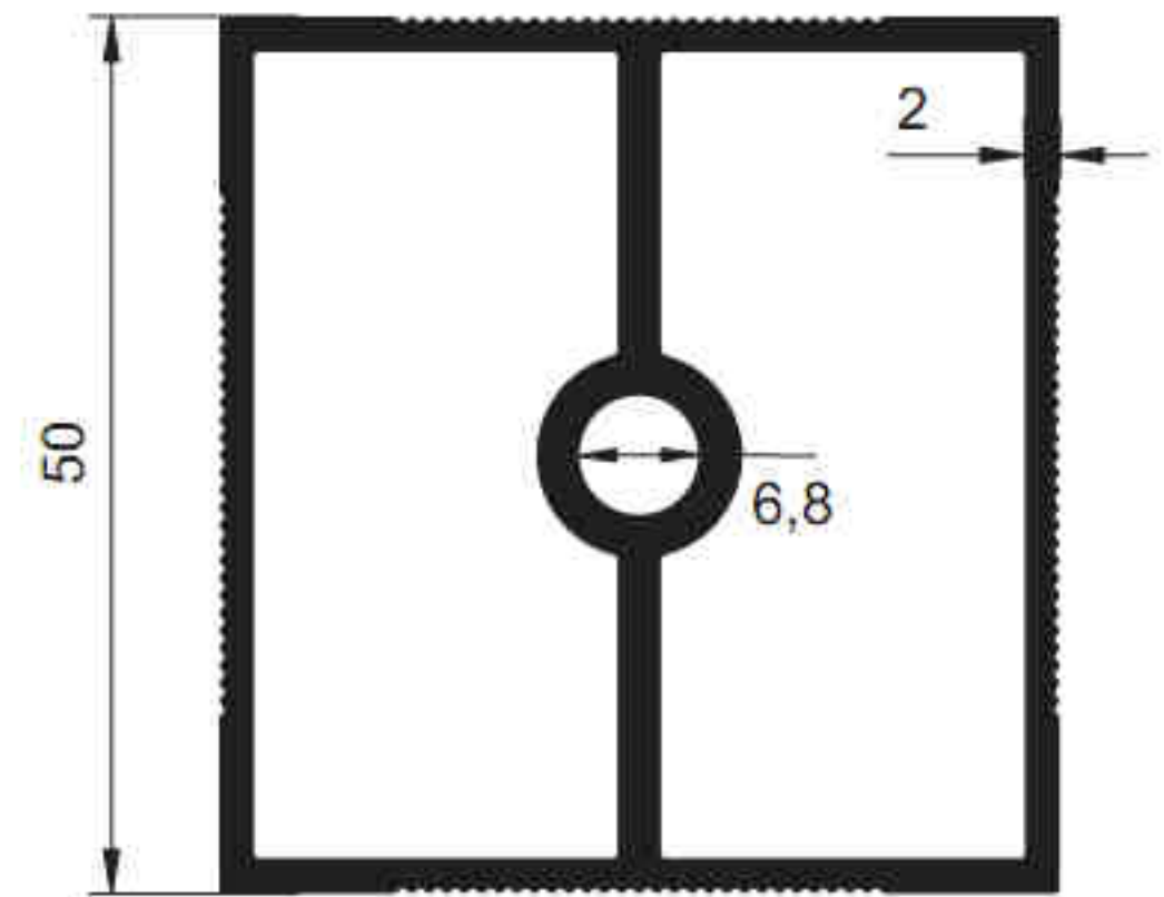
4685 - 1.398 kg/m
