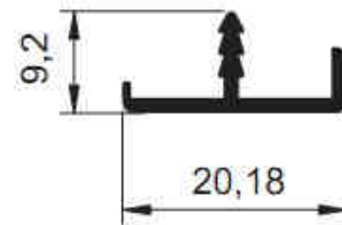
4258 - 0.132 kg/m
