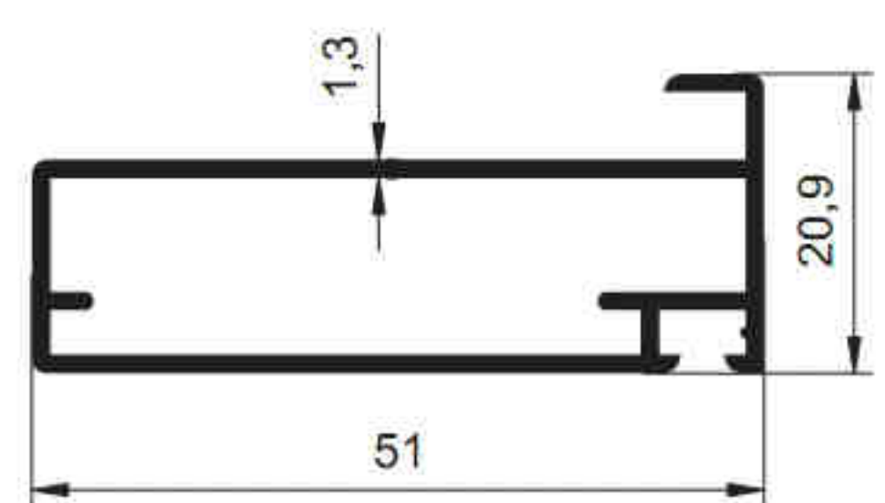
2022 - 0.527 kg/m
