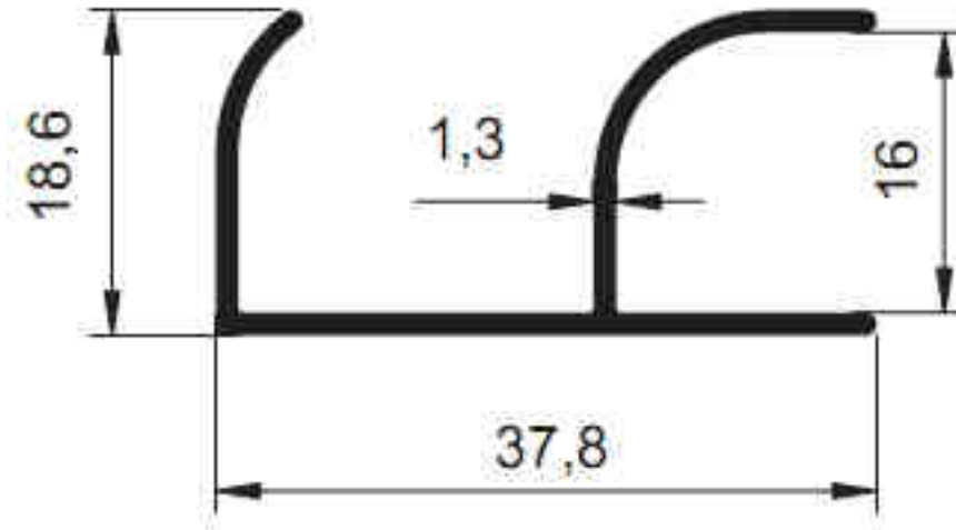
3390 - 0.295 kg/m
