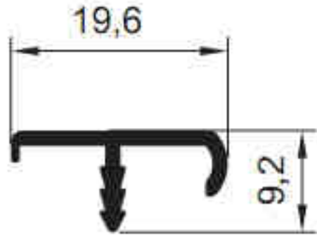
6203 - 0.128 kg/m
