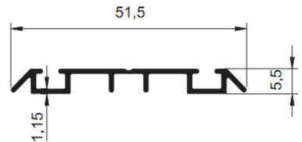
3393 - 0.267 kg/m
