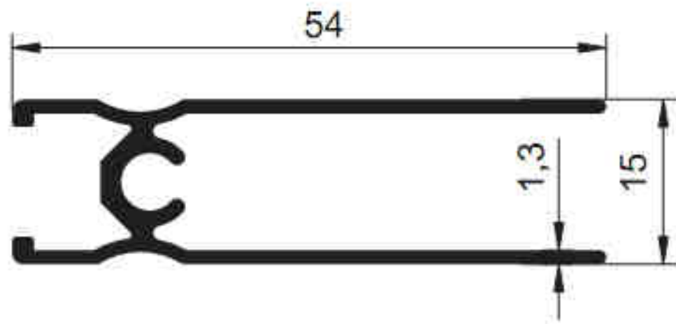
3541 - 0.490 kg/m
