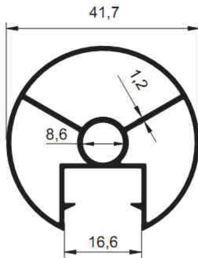
3537 - 0.657 kg/m
