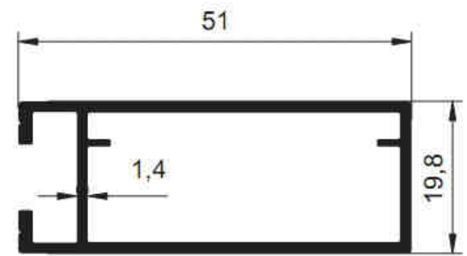
4807 - 0.599 kg/m
