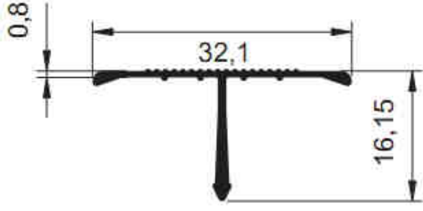
3778 - 0.148 kg/m
