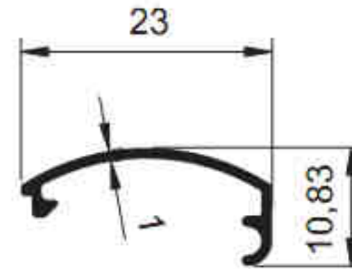
3665 - 0.103 kg/m
