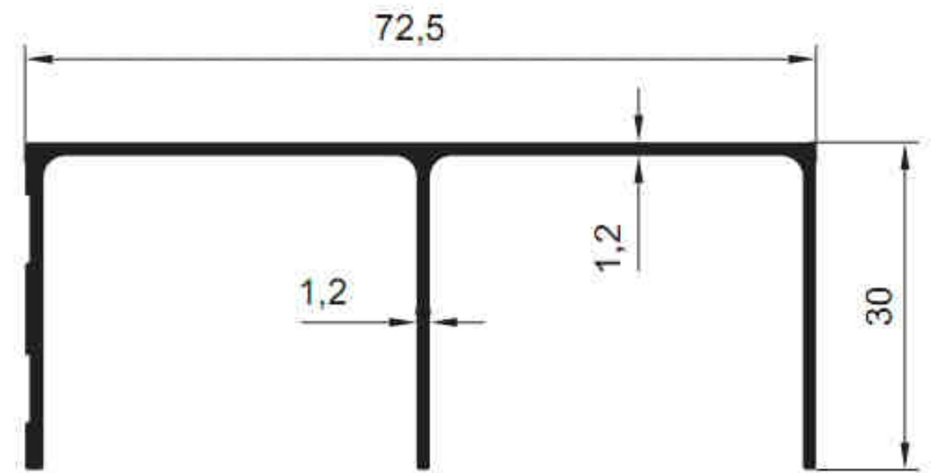
5541 - 0.550 kg/m
