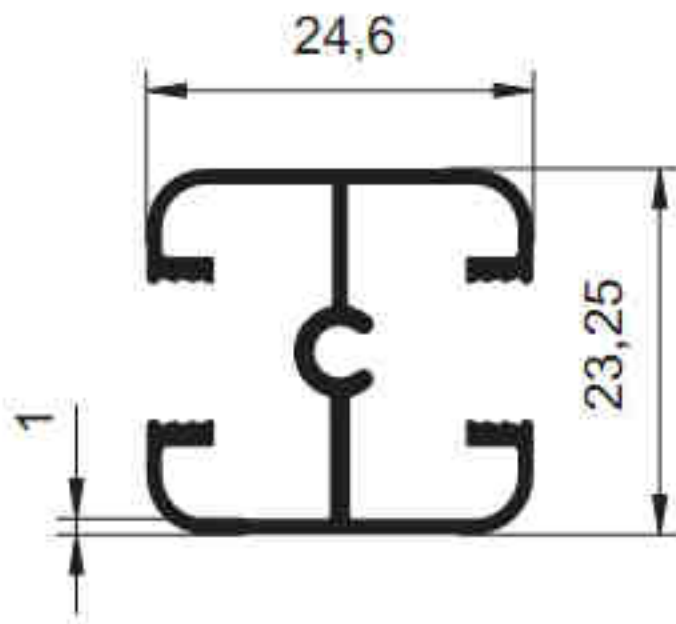
3671 - 0.331 kg/m
