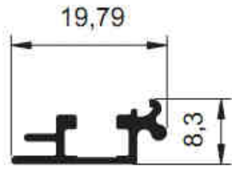
2919 - 0.131 kg/m
