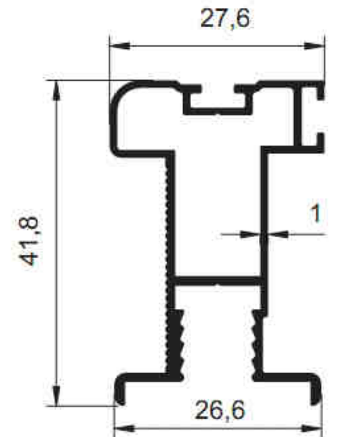
5058 - 0.500 kg/m
