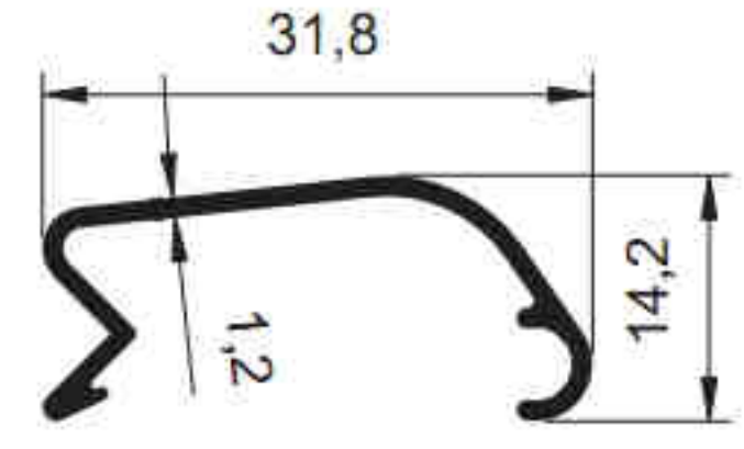
3286 - 0.264 kg/m
