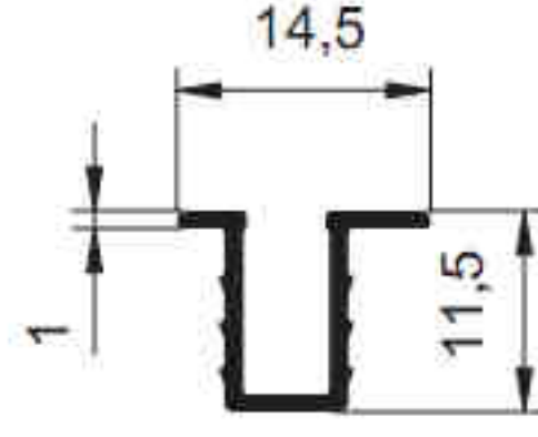
3956 - 0.105 kg/m
