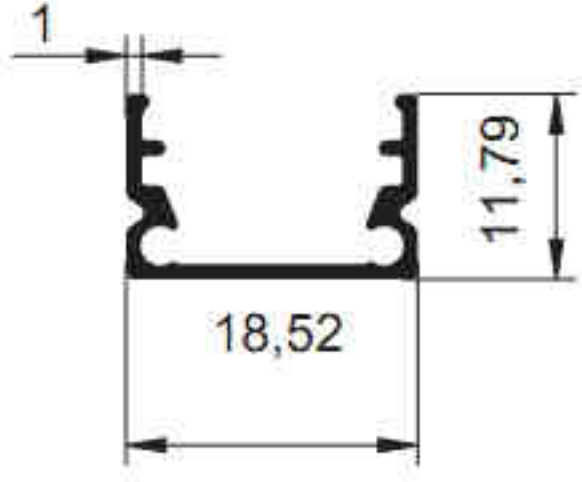
4950 - 0.139 kg/m
