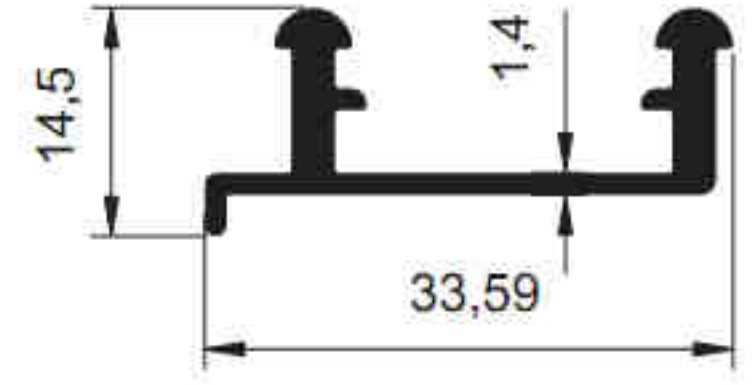
3954 - 0.320 kg/m
