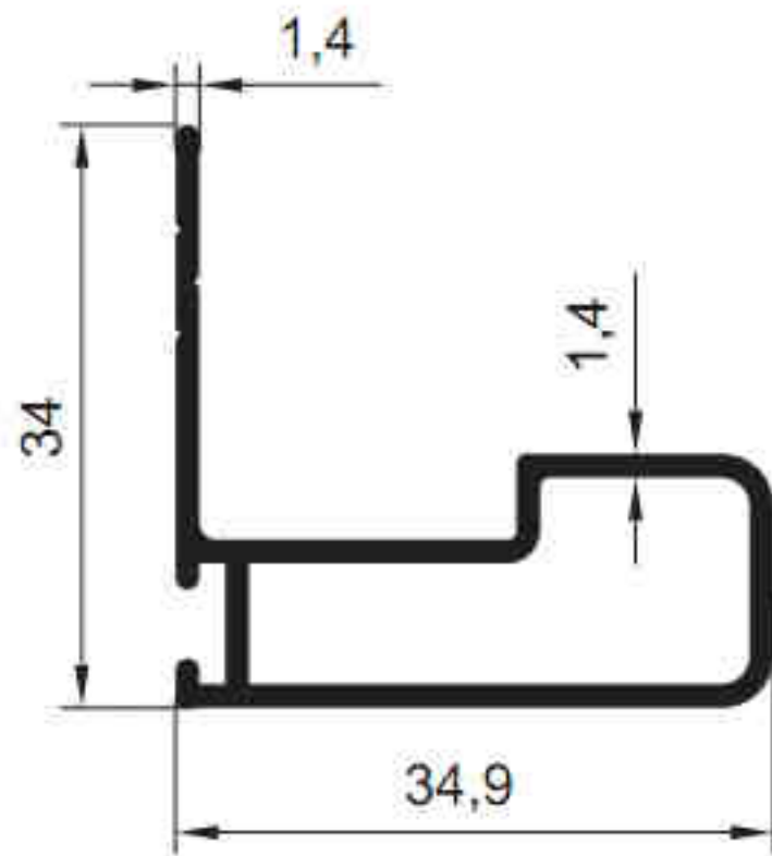
5735 - 0.447 kg/m
