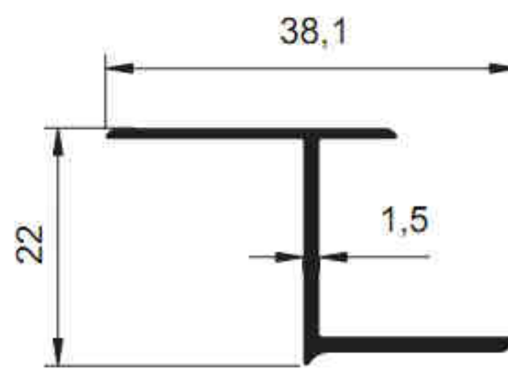
3459 - 0.227 kg/m
