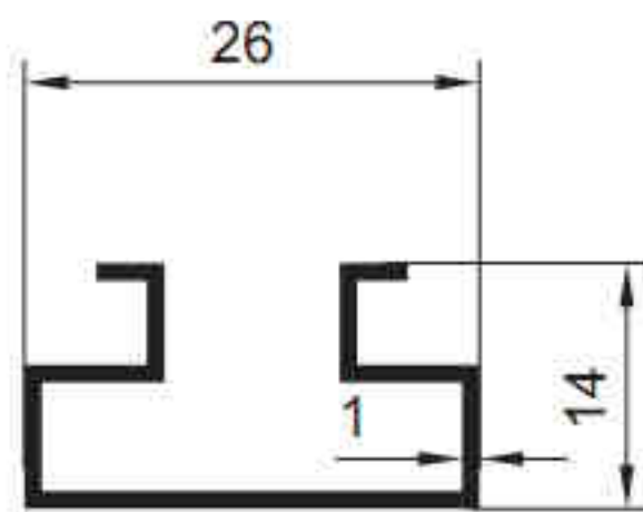
6230 - 0.195 kg/m
