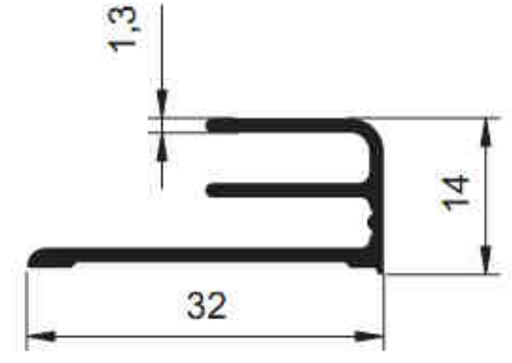
3957 - 0.262 kg/m
