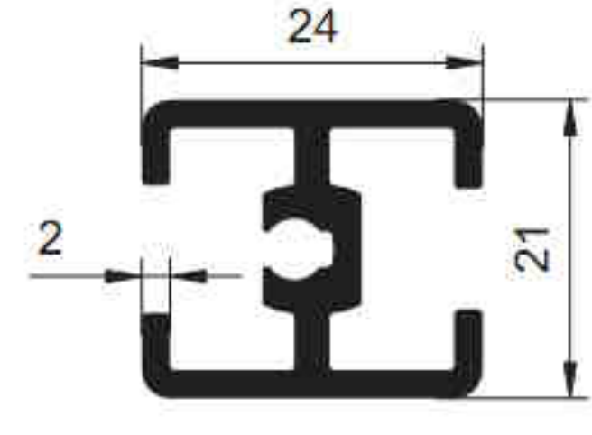
4249 - 0.513 kg/m
