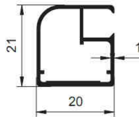
3631 - 0.257 kg/m
