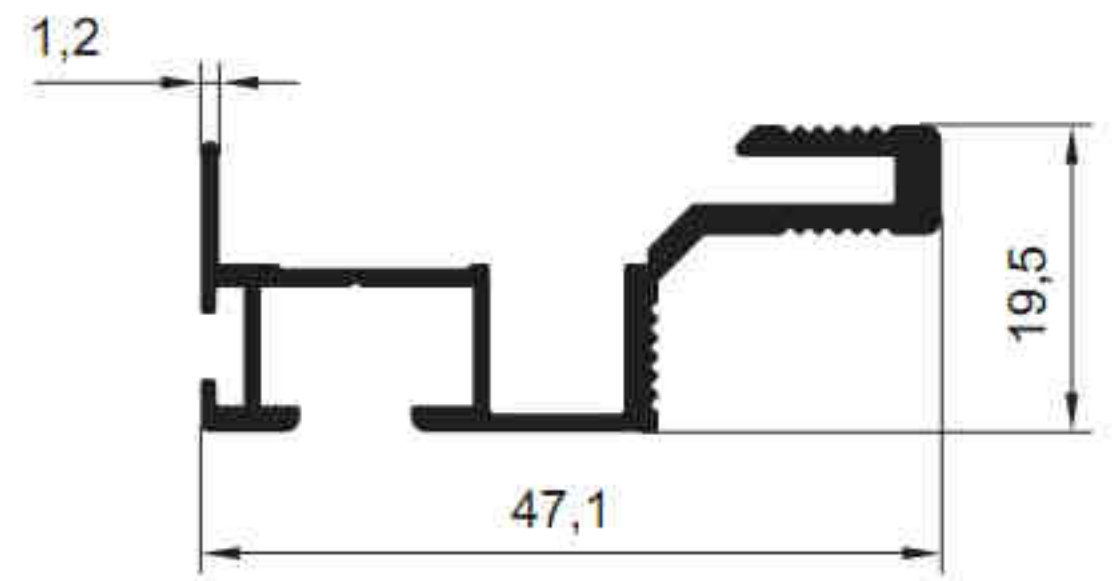
6092 - 0.470 kg/m
