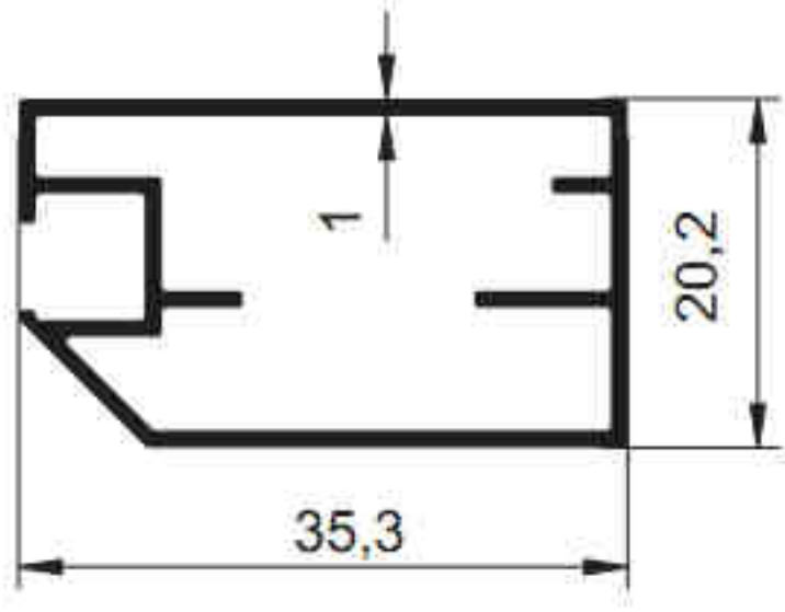
3774 - 0.364 kg/m
