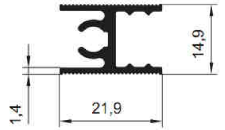
5727 - 0.296 kg/m
