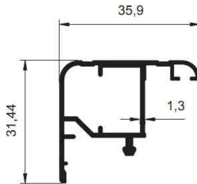
5027 - 0.470 kg/m
