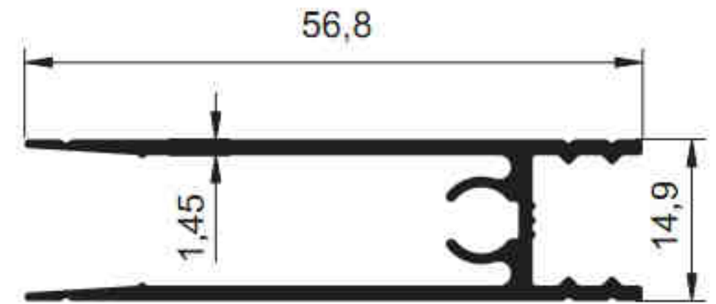
4426 - 0.535 kg/m
