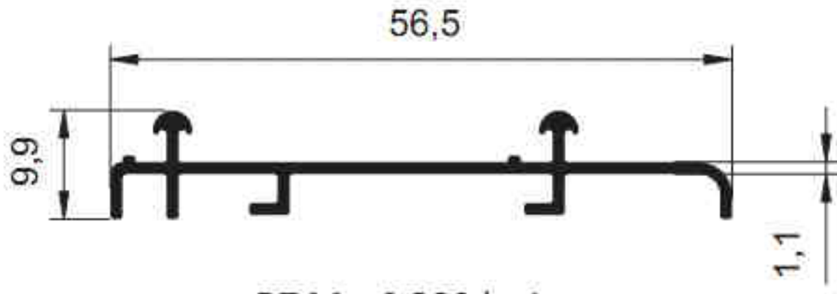
3711 - 0.289 kg/m
