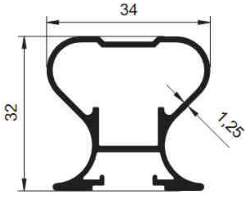
3478 - 0.527 kg/m
