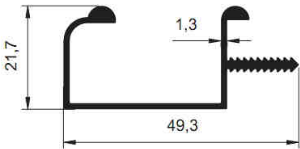
5123 - 0.437 kg/m
