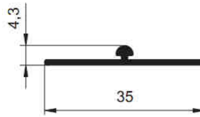
5026 - 0.136 kg/m
