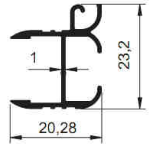
4837 - 0.239 kg/m
