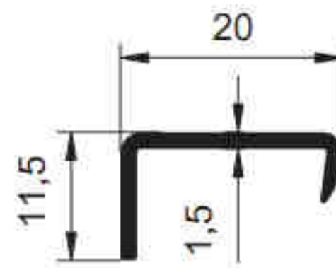
3404 - 0.135 kg/m
