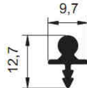
3394 - 0.124 kg/m
