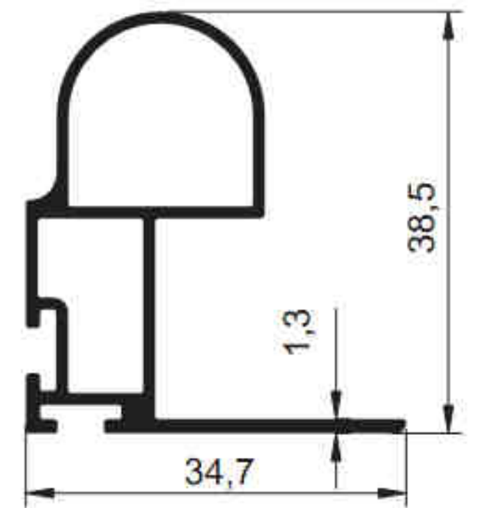
3406 - 0.477 kg/m
