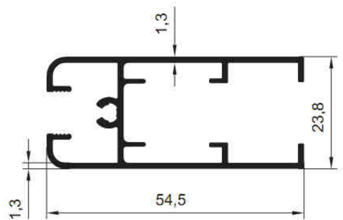
5955 - 0.656 kg/m
