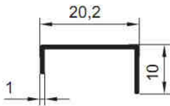
5844 - 0.092 kg/m
