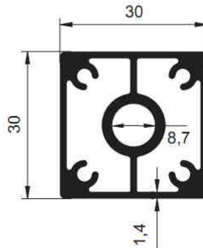
4027 - 0.934 kg/m
