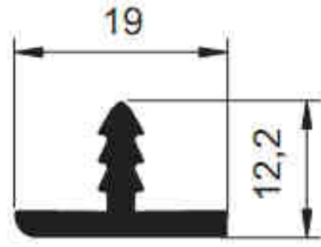
3689 - 0.201 kg/m
