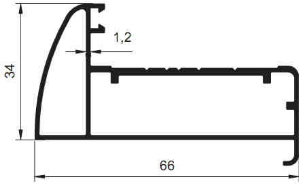
4420 - 0.840 kg/m
