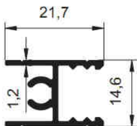
3472 - 0.249 kg/m
