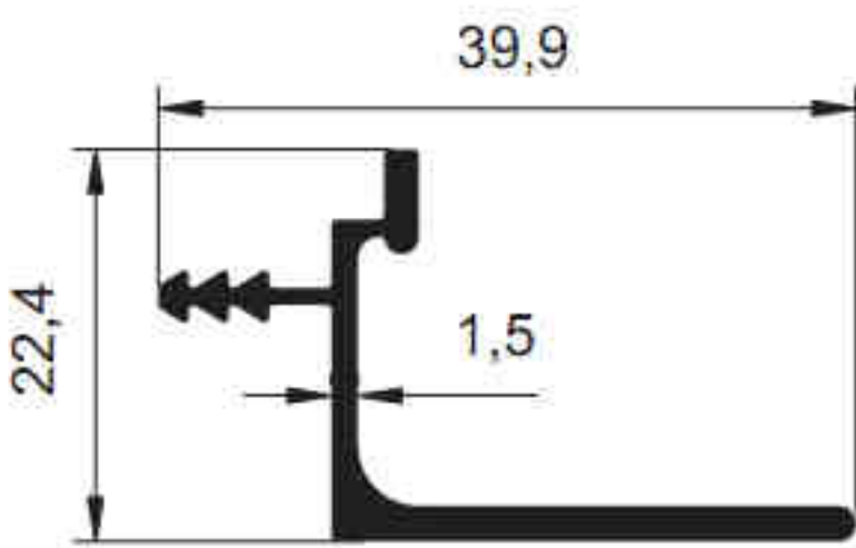
4031 - 0.318 kg/m
