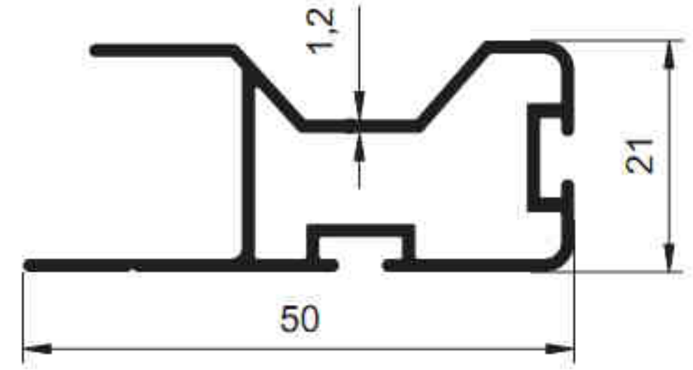
5199 - 0.497 kg/m
