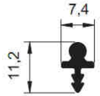
3395 - 0.098 kg/m
