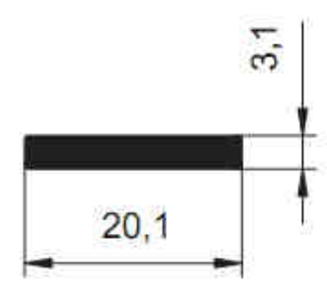
4989 - 0.168 kg/m
