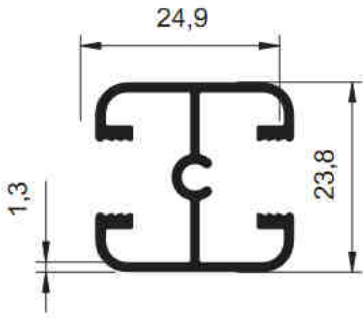
3522 - 0.399 kg/m
