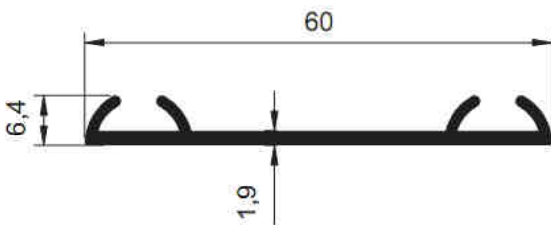
3398 - 0.396 kg/m
