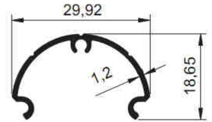
4281 - 0.204 kg/m
