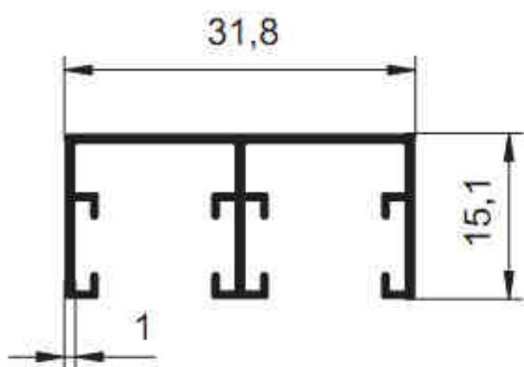
5213 - 0.266 kg/m
