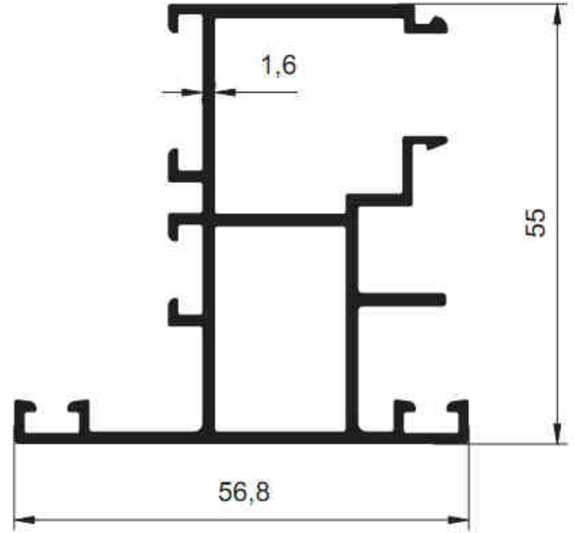
3145 - 1.108 kg/m
