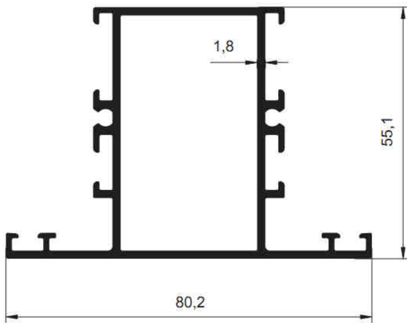
3140 - 1.381 kg/m
