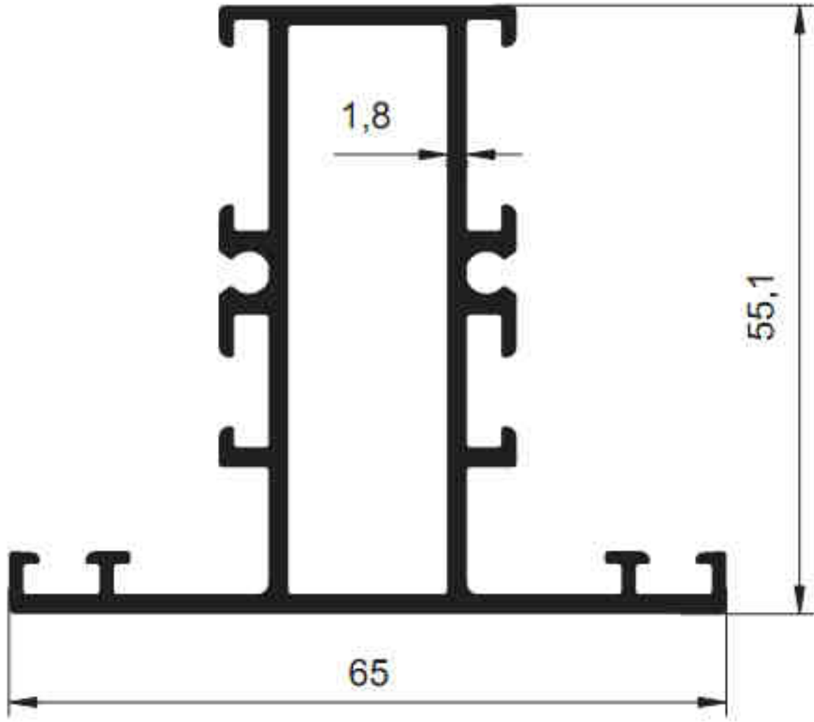
3256 - 1.244 kg/m
