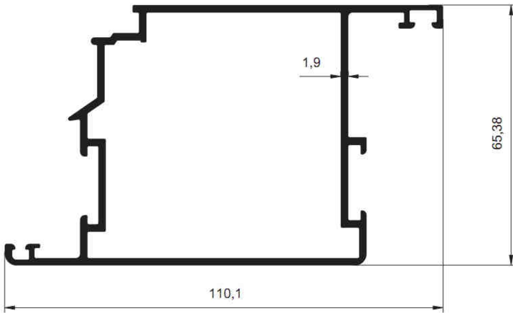
3144 - 1.788 kg/m
