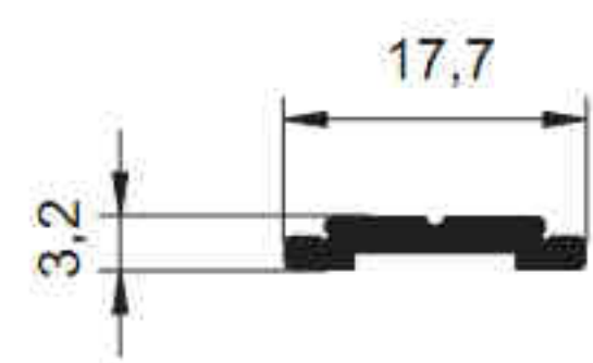
2790 - 0.149 kg/m
