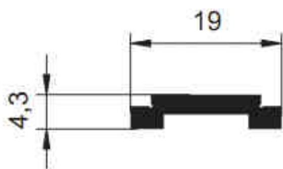
1523 - 0.149 kg/m
