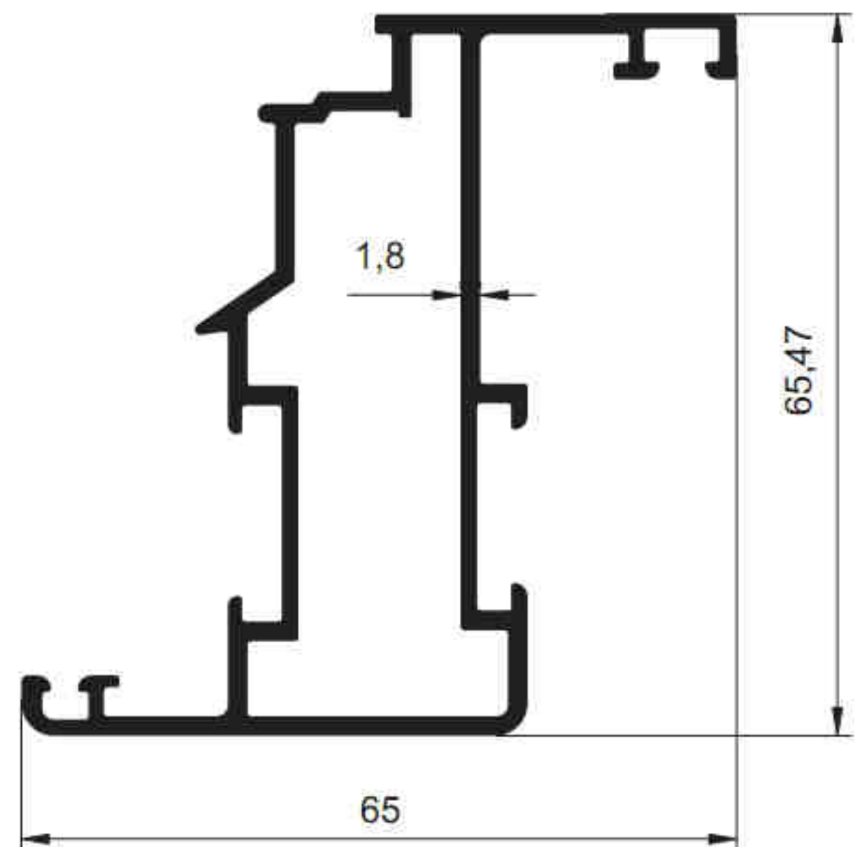
3258 - 1.229 kg/m
