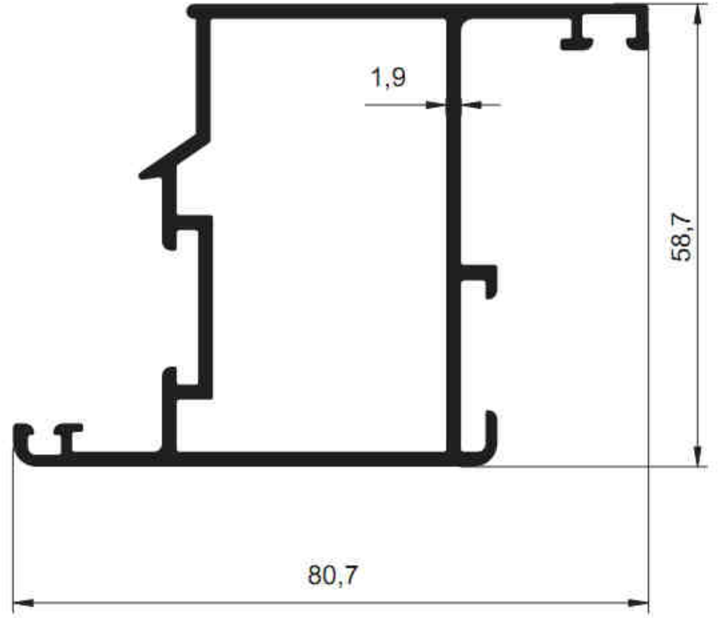
3143 - 1.396 kg/m
