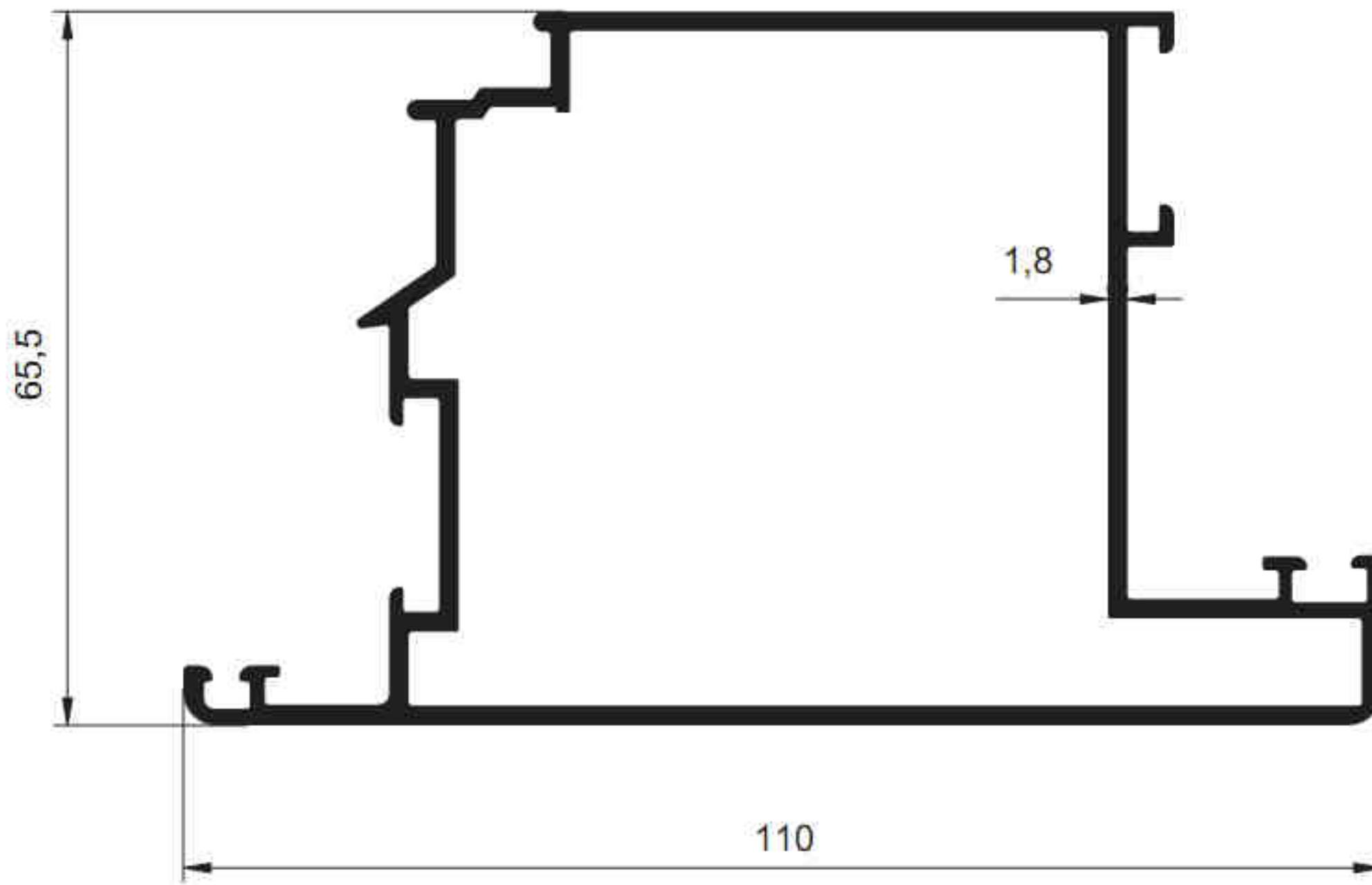
3342 - 1.781 kg/m
