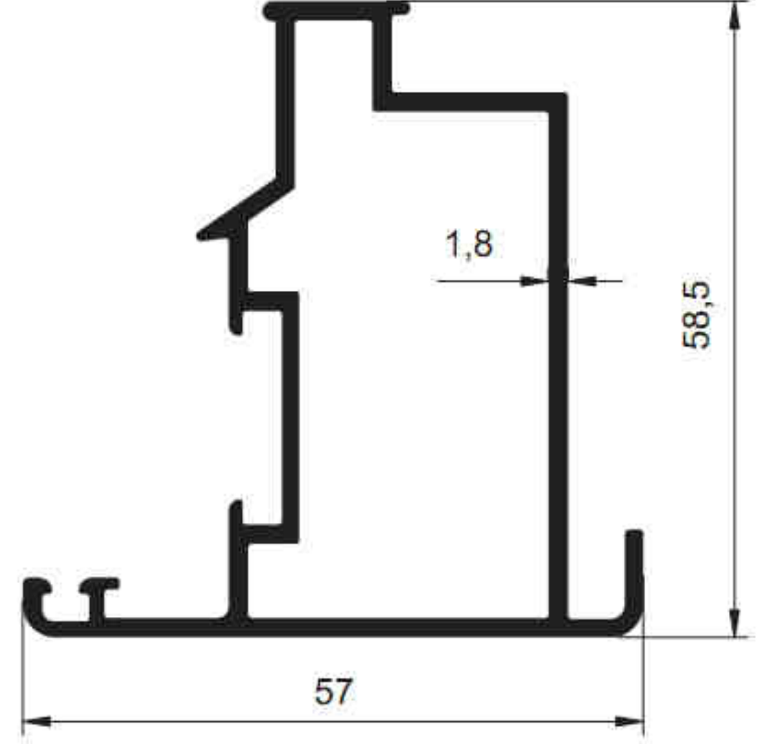
3341 - 1.093 kg/m
