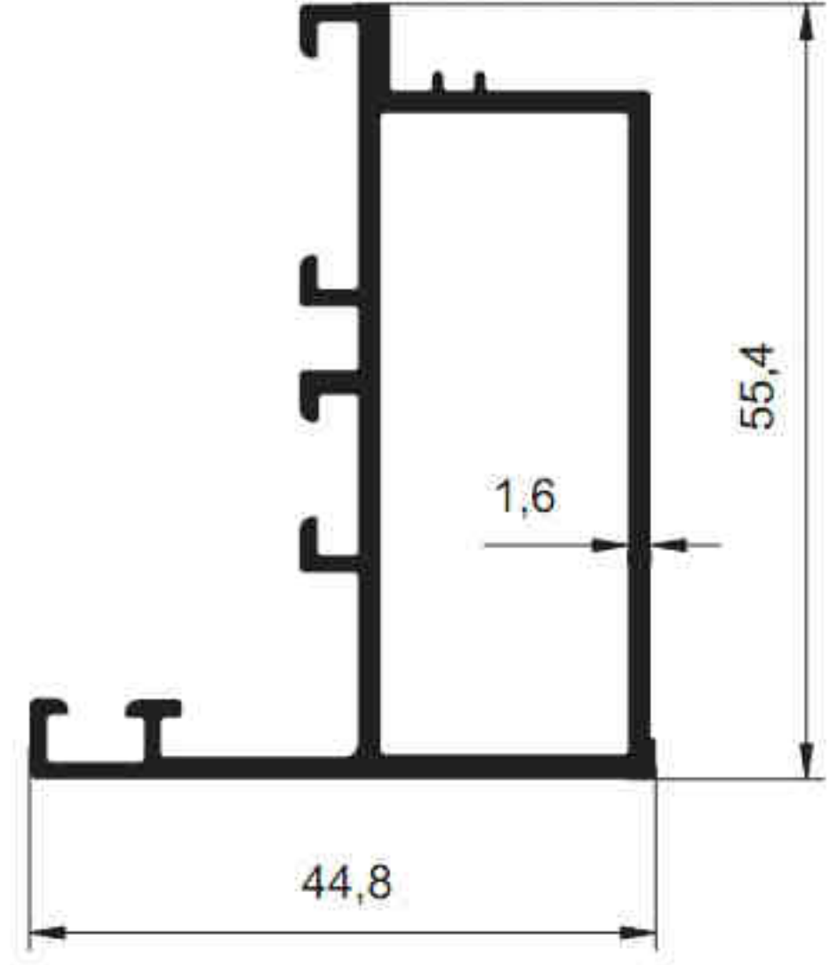
3338 - 0.866 kg/m
