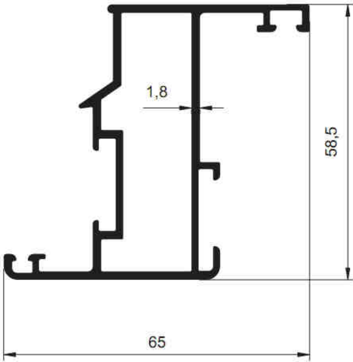
3259 - 1.142 kg/m
