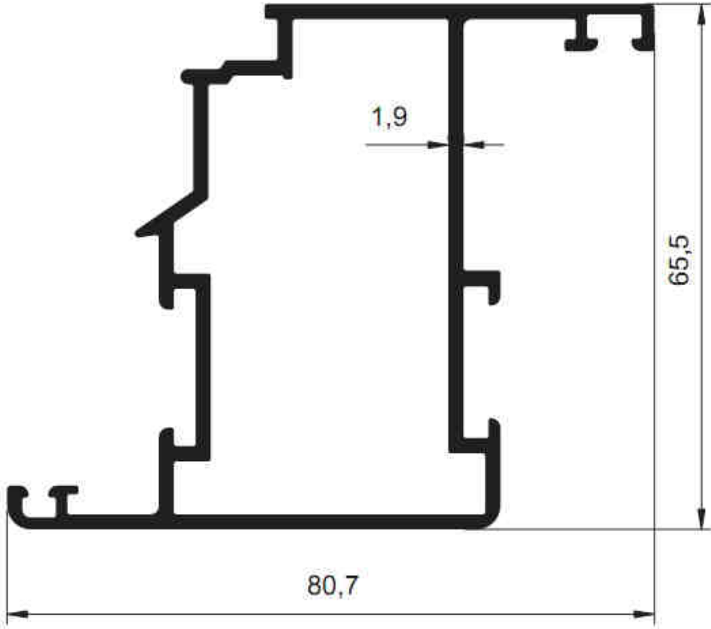
3139 - 1.486 kg/m
