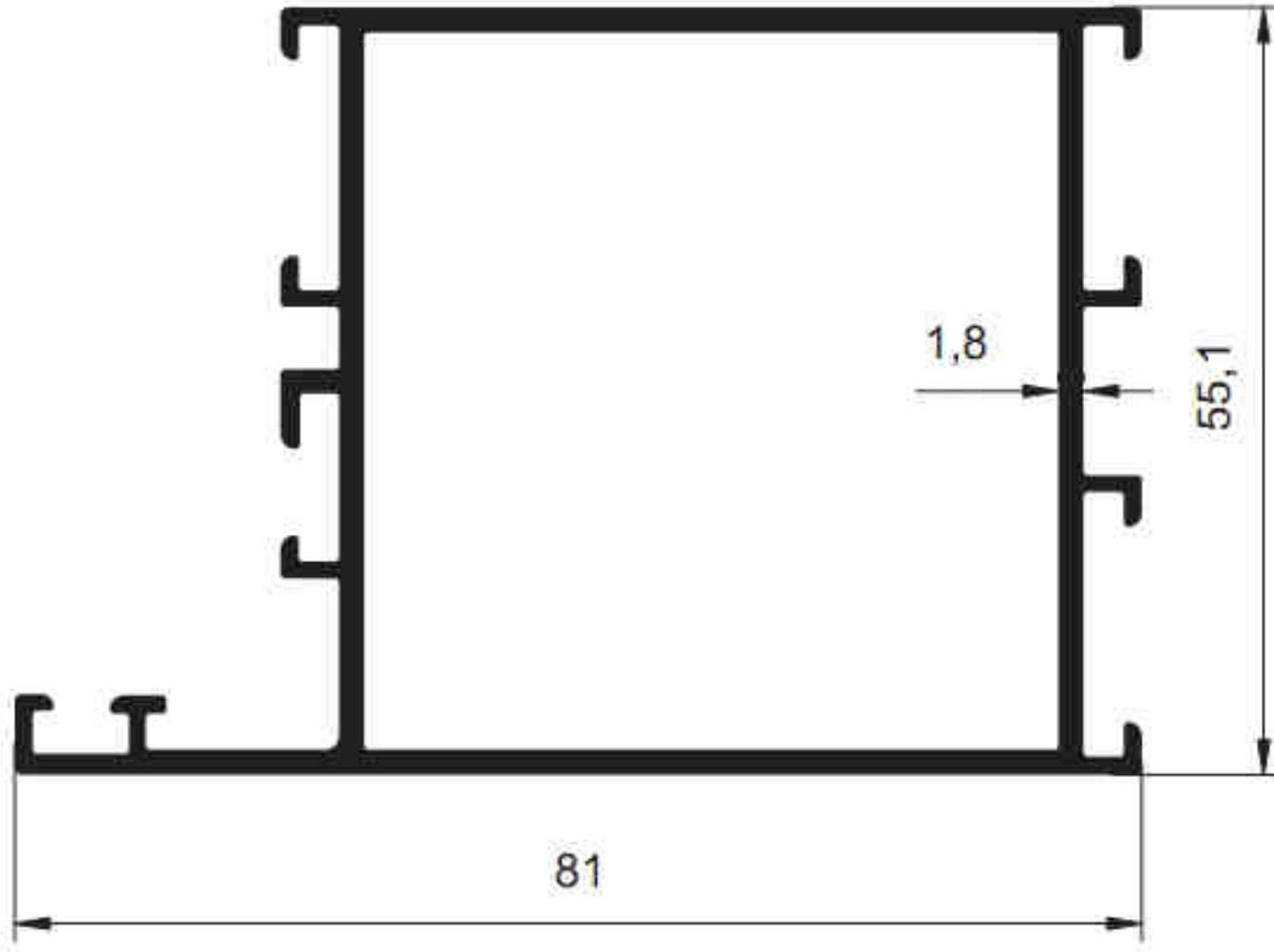
3340 - 1.357 kg/m
