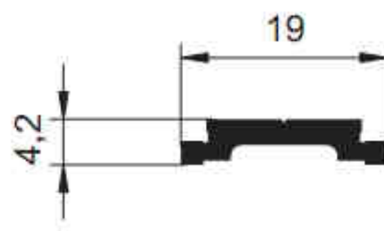
5254 - 0.138 kg/m
