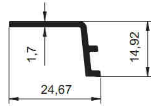
3000 - 0.177 kg/m
