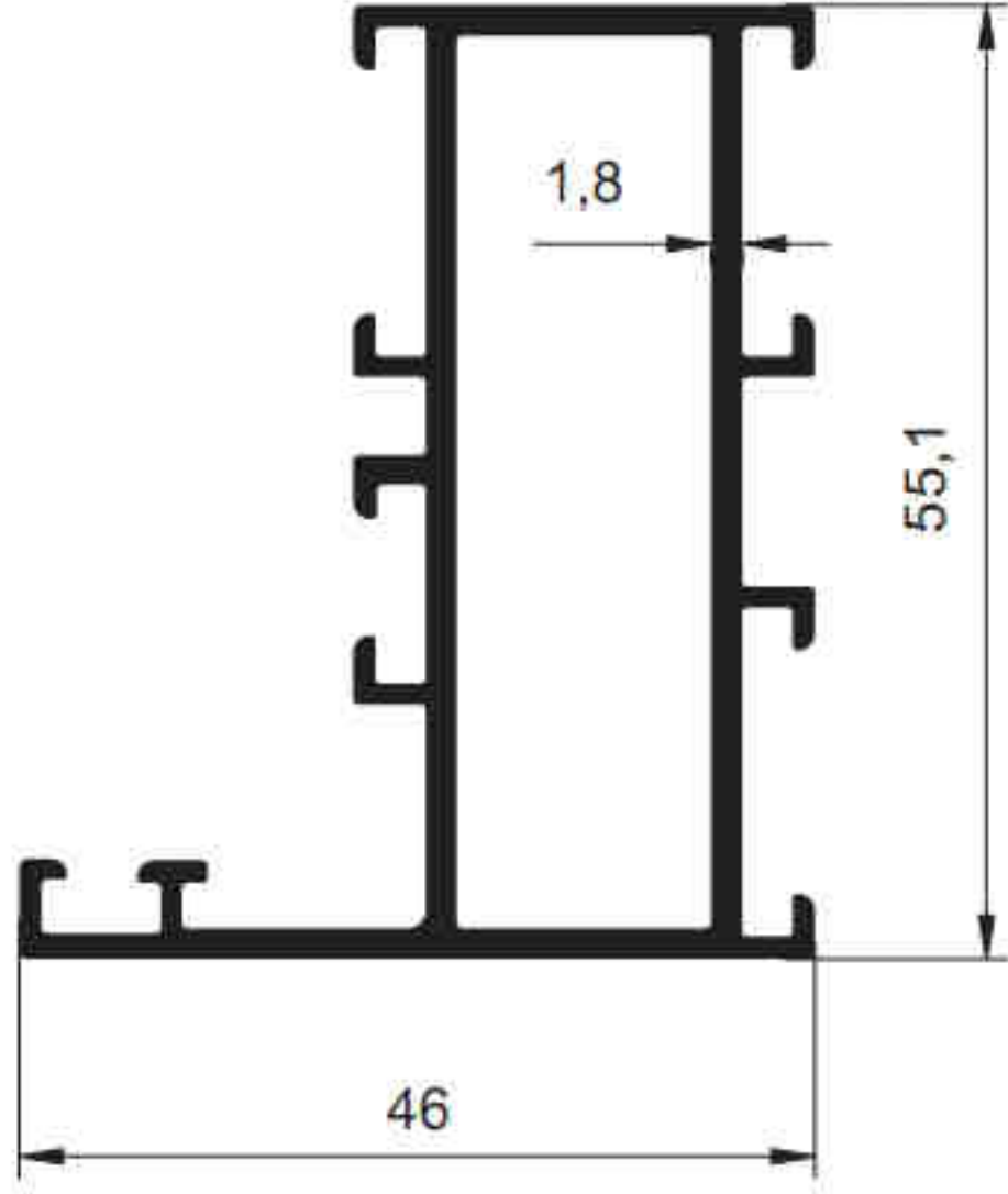
3339 - 1.012 kg/m
