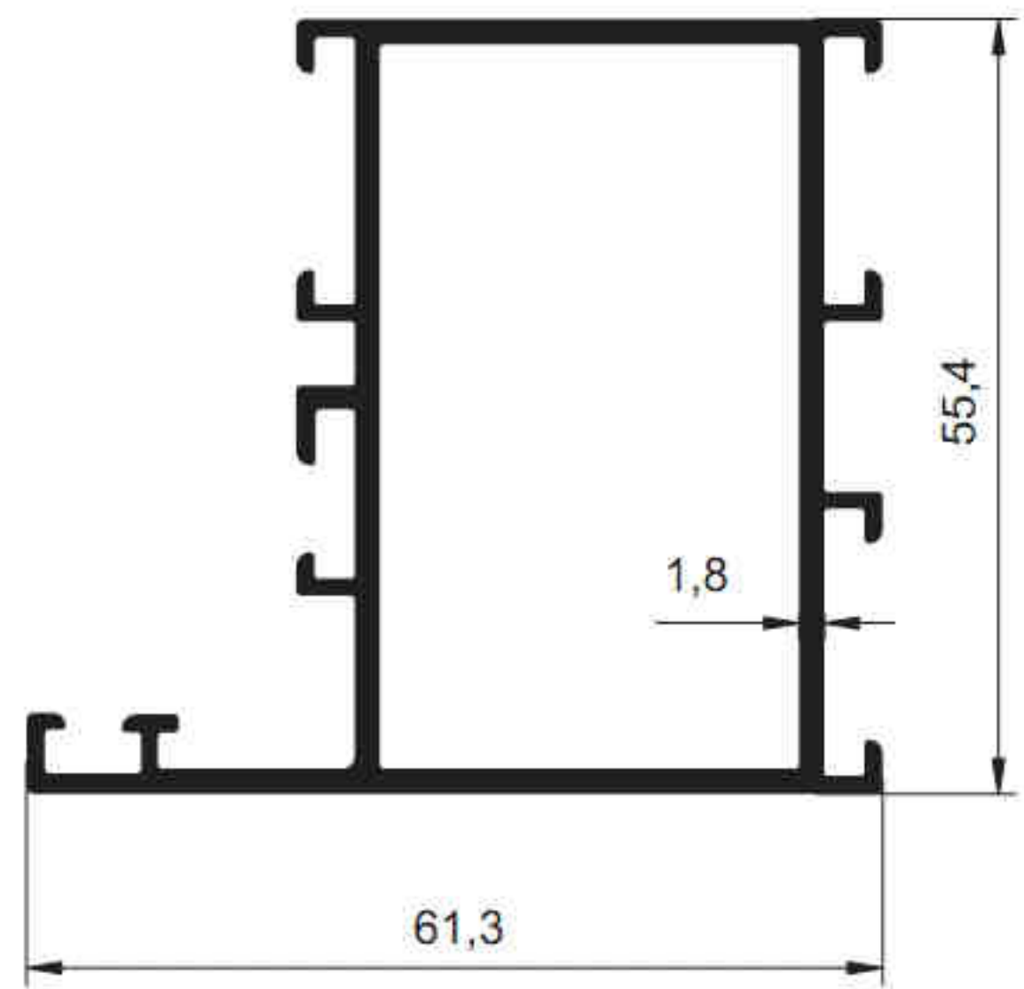
3142 - 1.169 kg/m
