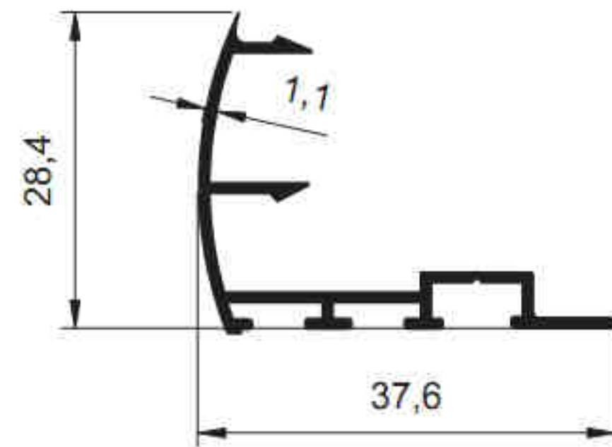
2149 - 0.304 kg/m
