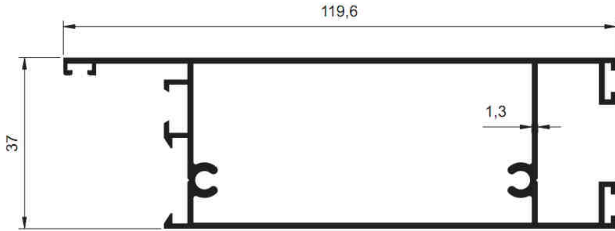
2168 - 1.291 kg/m
