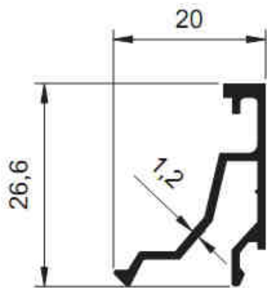
2151 - 0.218 kg/m
