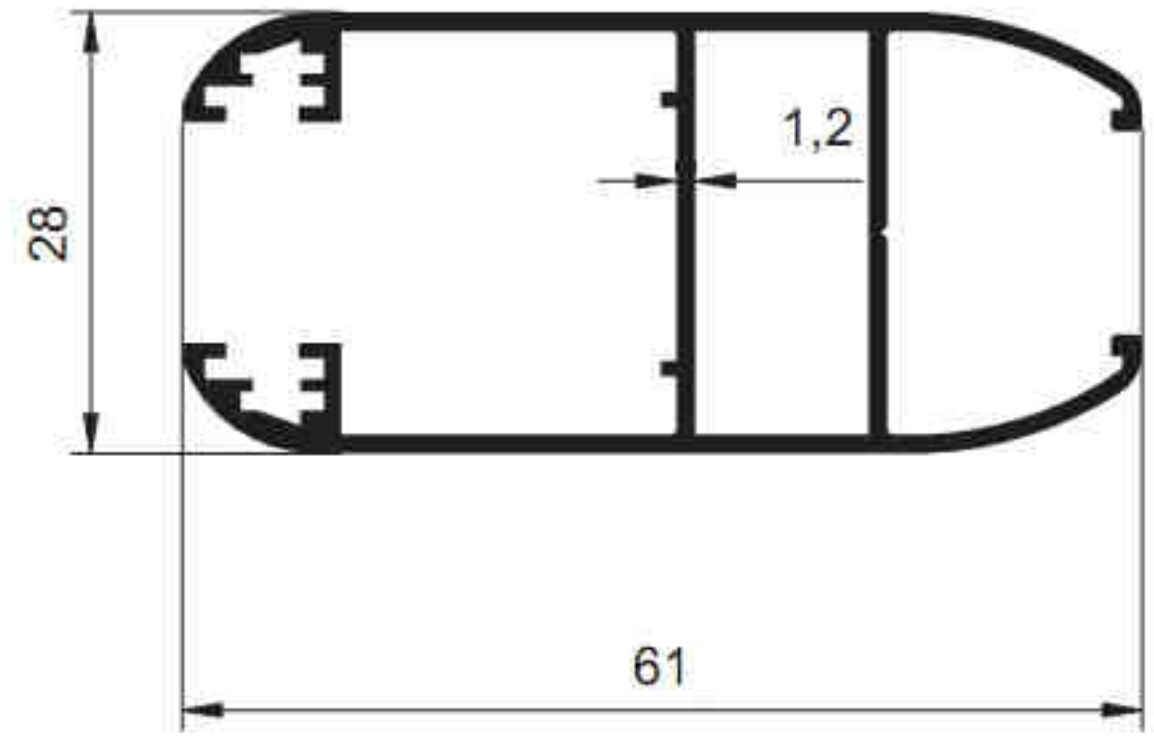
2155 - 0.701 kg/m
