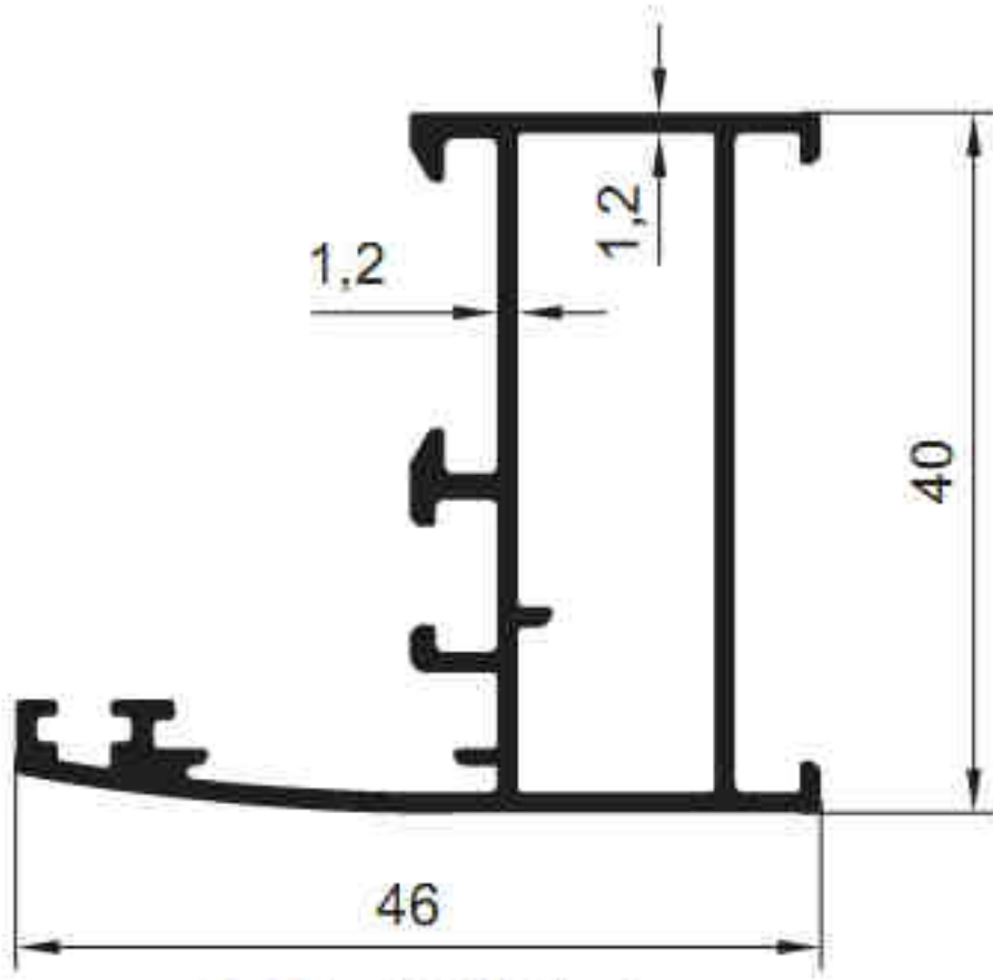
6003 - 0.622 kg/m
