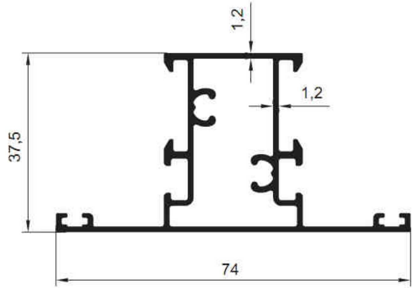
6006 - 0.845 kg/m
