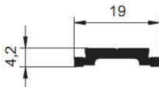
5254 - 0.138 kg/m
