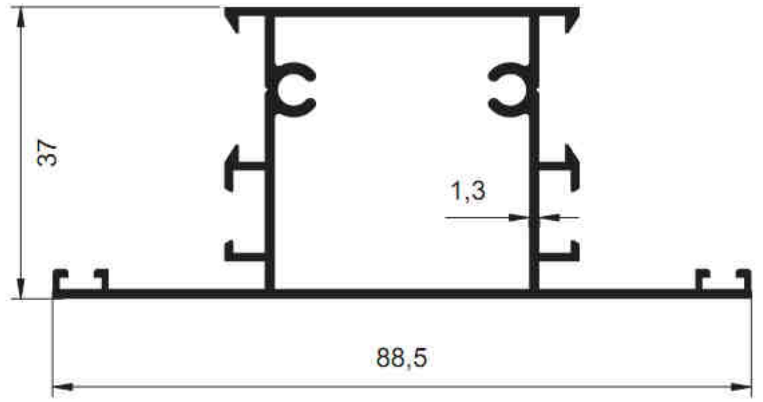
2158 - 0.950 kg/m
