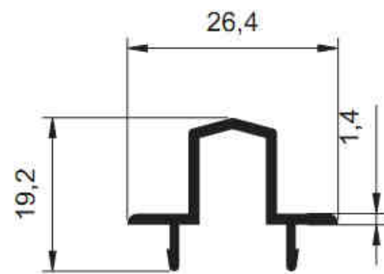
2428 - 0.220 kg/m
