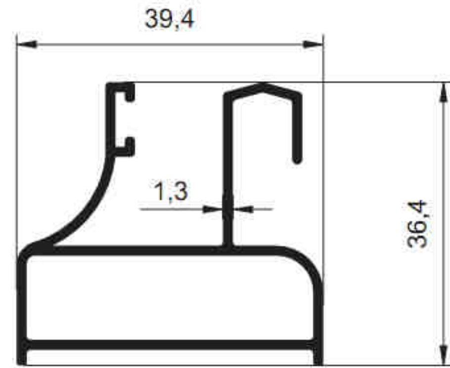
2427 - 0.600 kg/m
