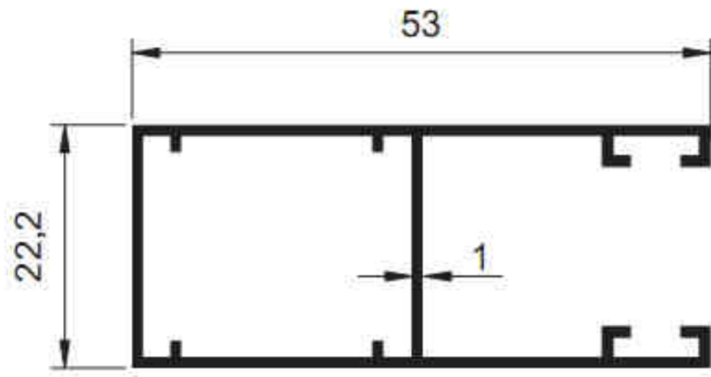
2169 - 0.465 kg/m
