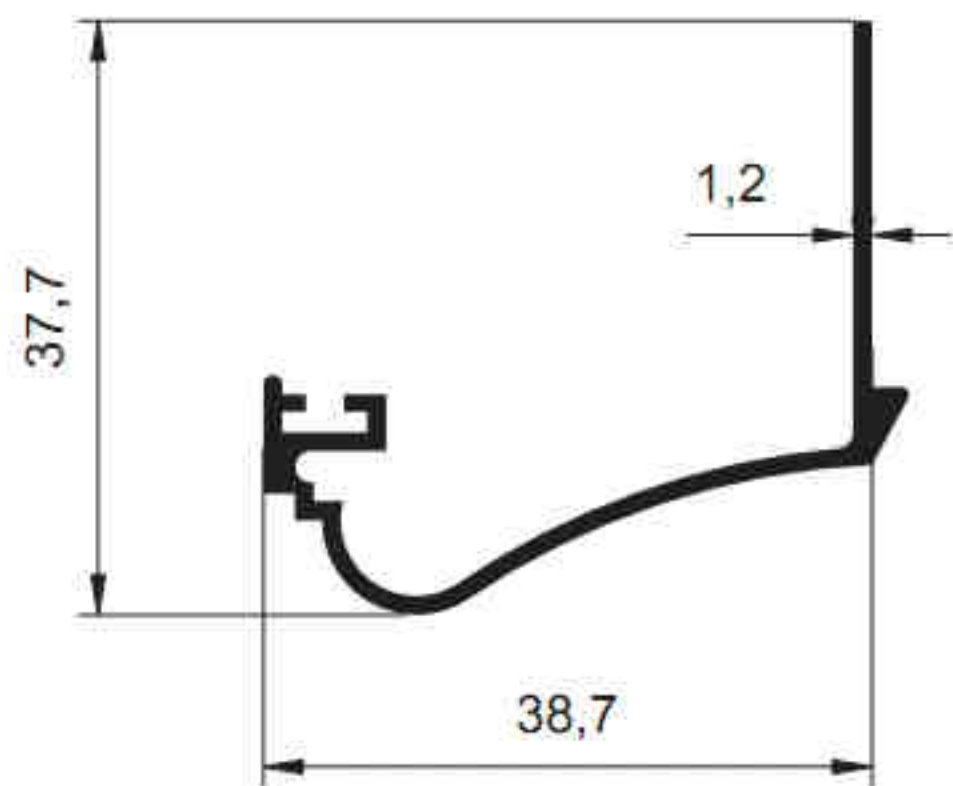
2216 - 0.316 kg/m
