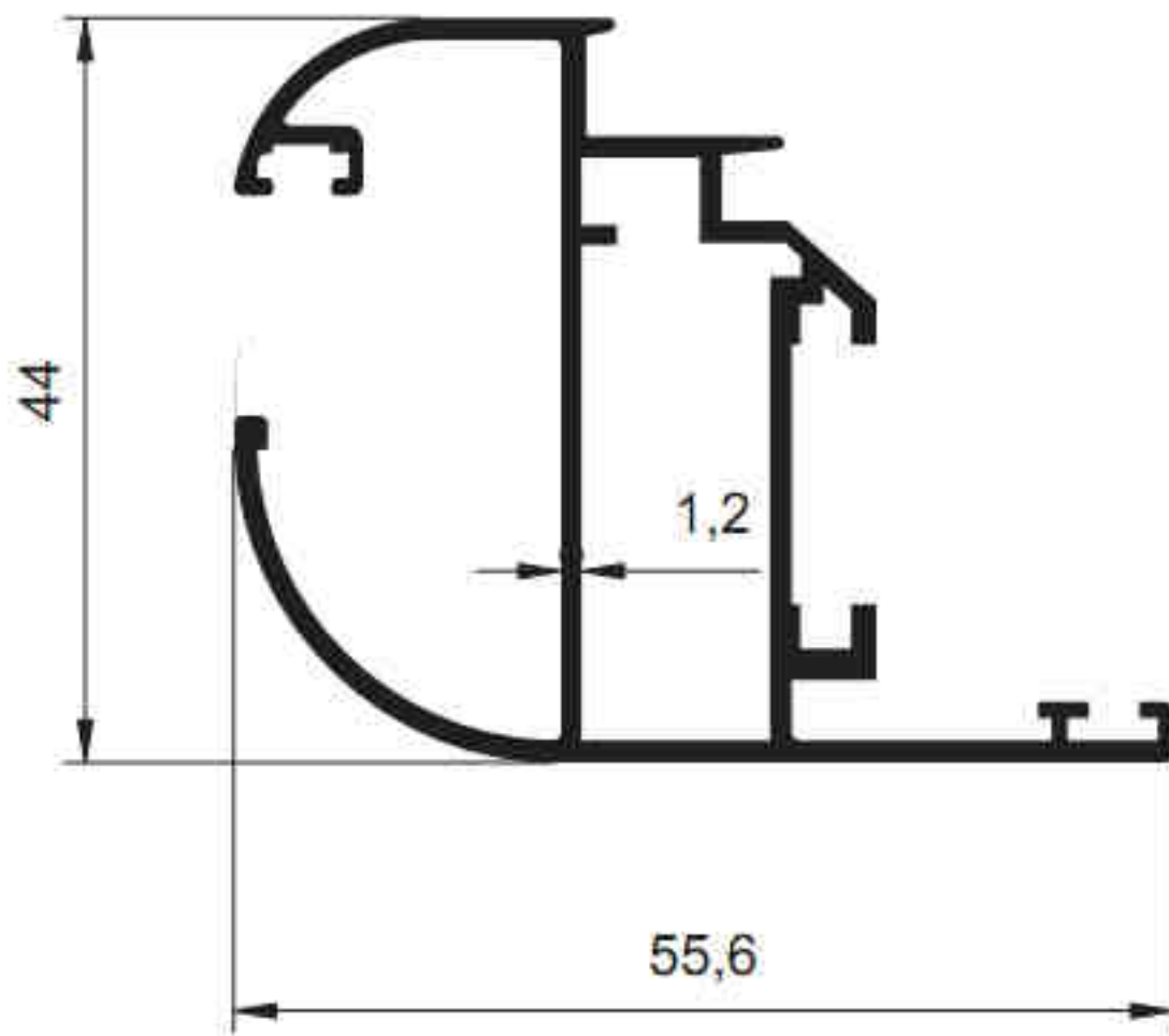
2223 - 0.779 kg/m
