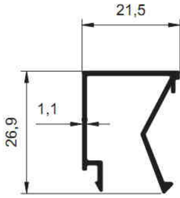
2148 - 0.262 kg/m
