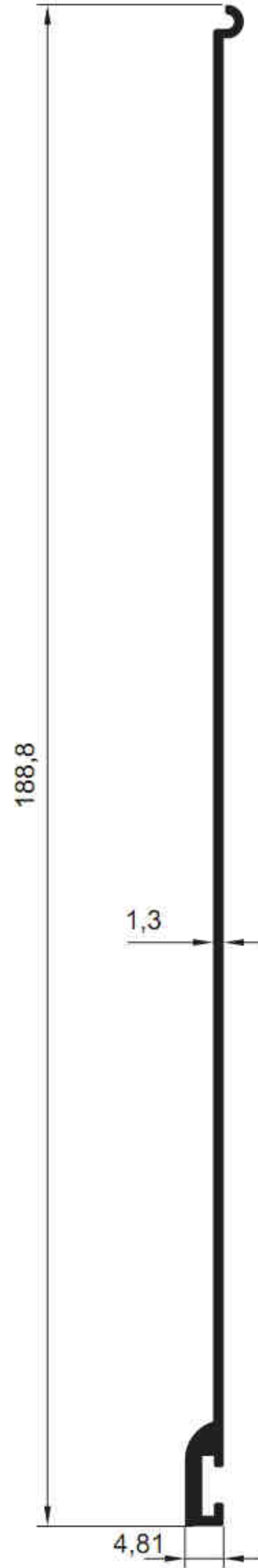
5582 - 0.737 kg/m
