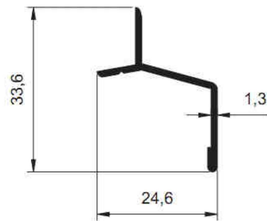
2145 - 0.193 kg/m
