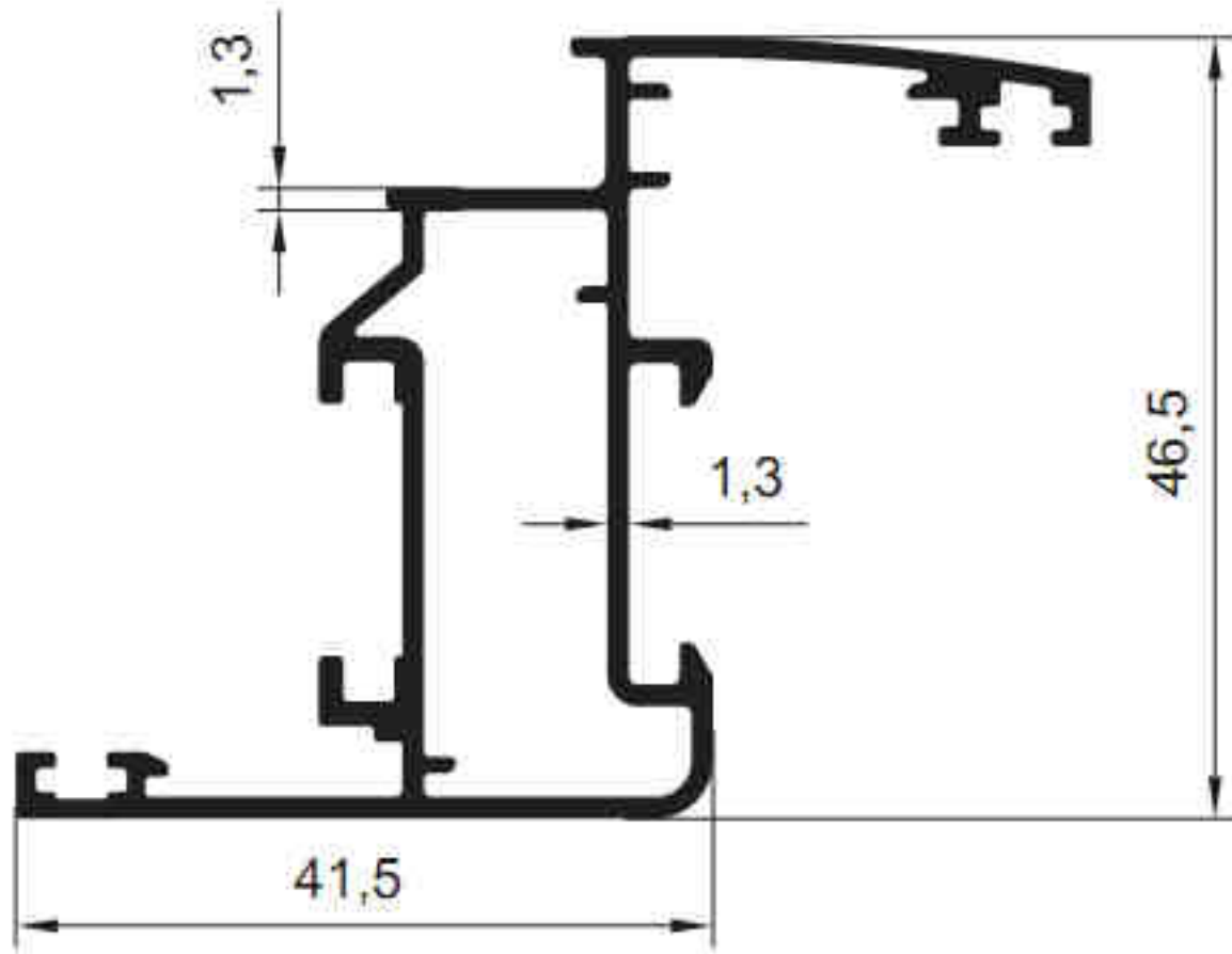
6005 - 0.812 kg/m
