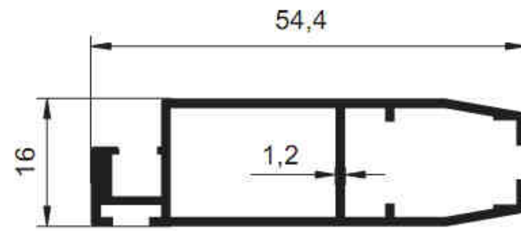
2202 - 0.513 kg/m
