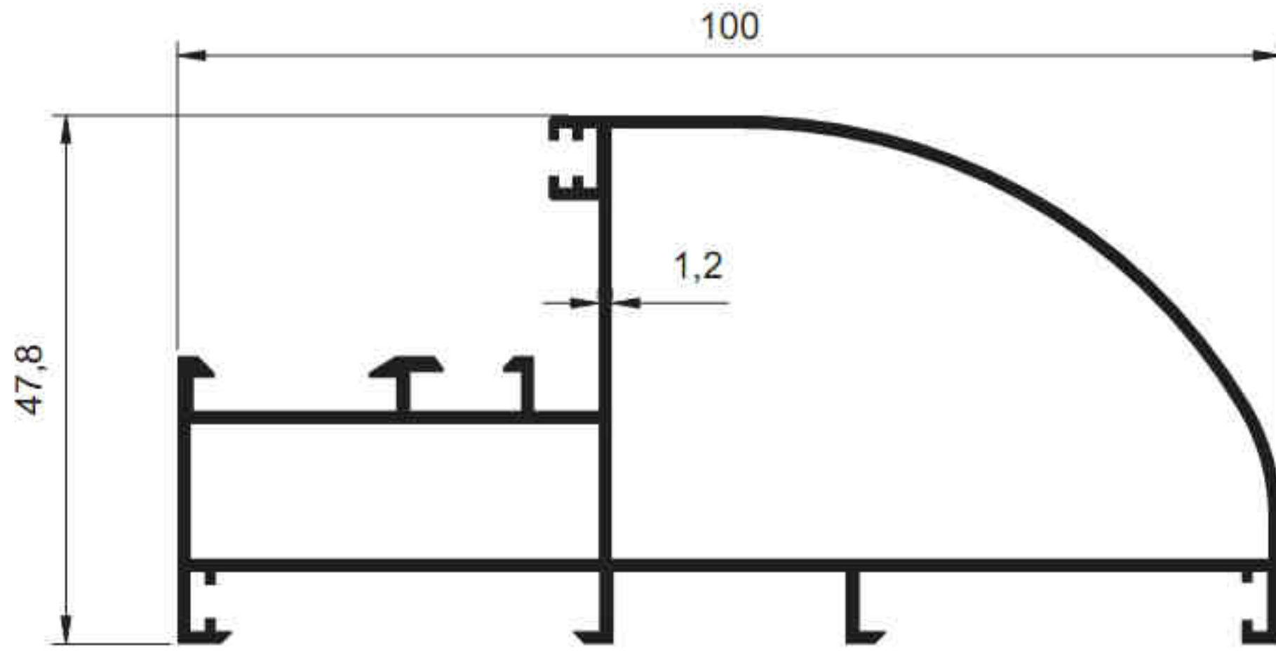
2348 - 1.138 kg/m
