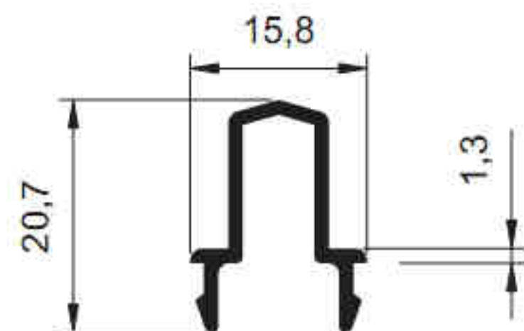
2225 - 0.189 kg/m
