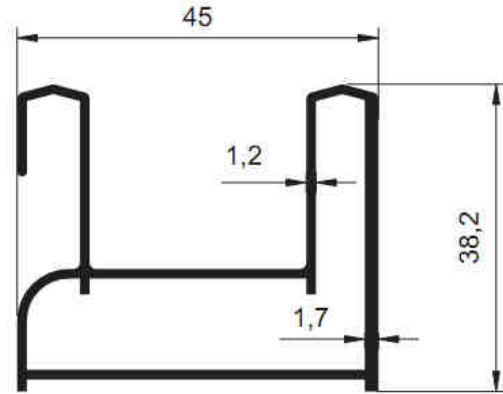
2164 - 0.697 kg/m
