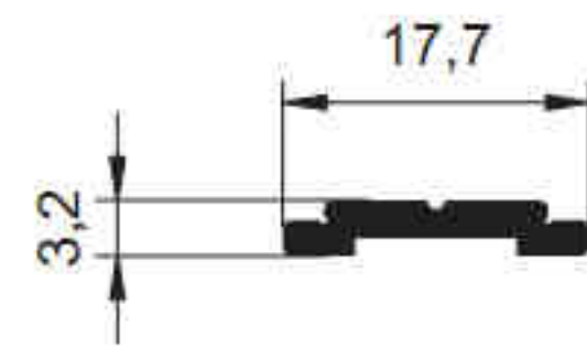
2790 - 0.111 kg/m
