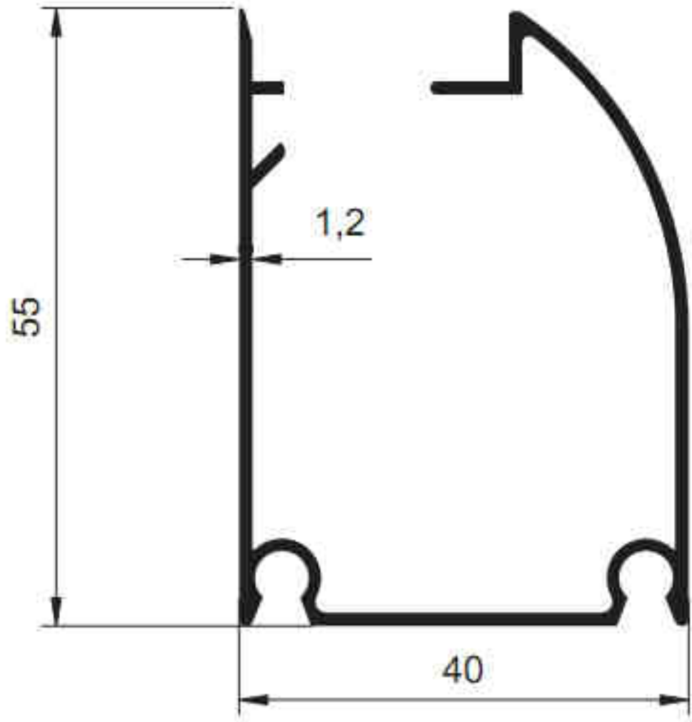
2119 - 0.599 kg/m
