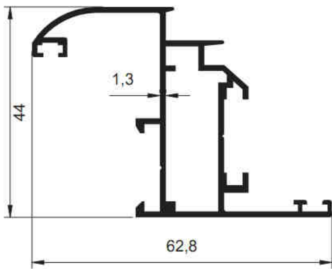
2162 - 0.729 kg/m
