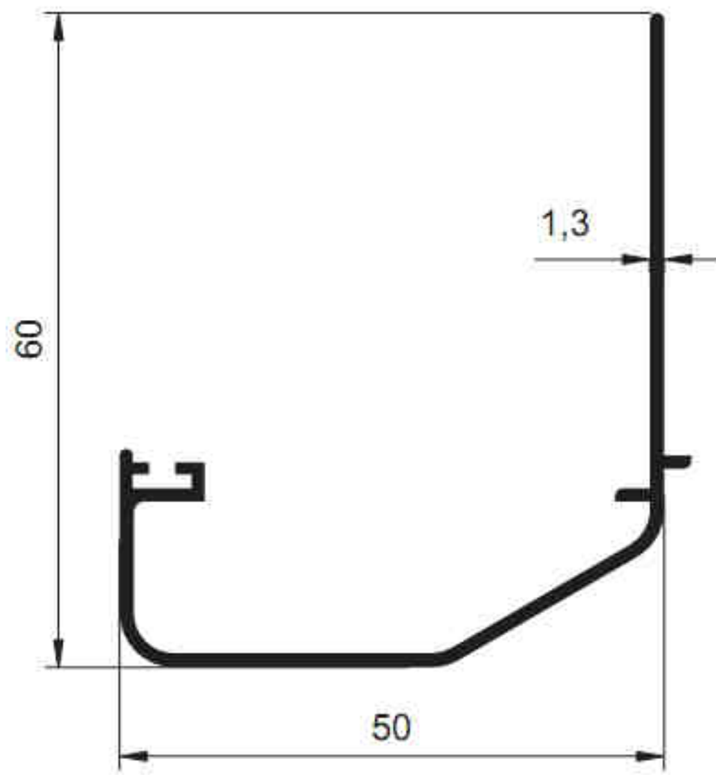
2215 - 0.464 kg/m
