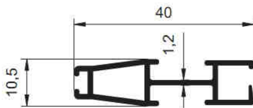
2224 - 0.327 kg/m
