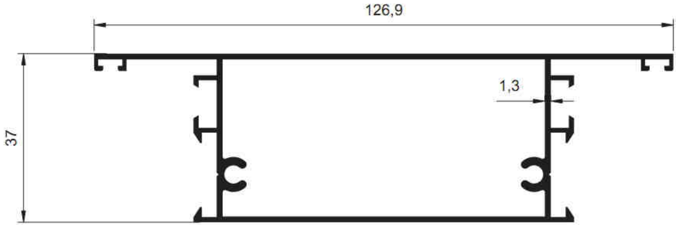
2167 - 1.239 kg/m
