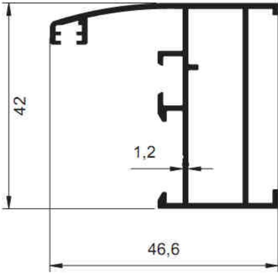
2147 - 0.608 kg/m
