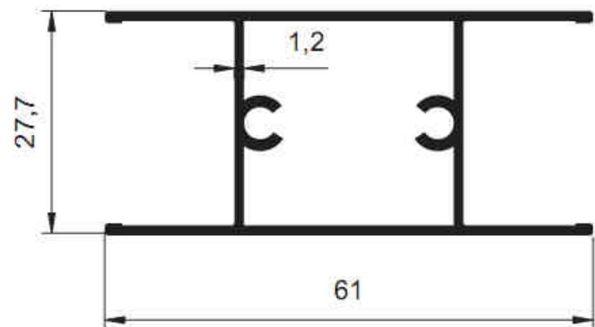
2146 - 0.662 kg/m
