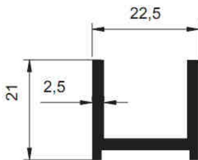
2249 - 0.396 kg/m
