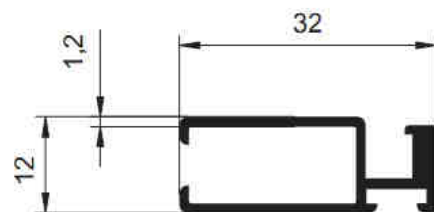
2156 - 0.300 kg/m
