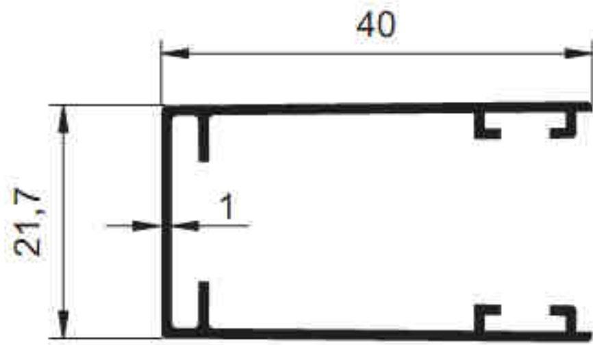
2217 - 0.335 kg/m
