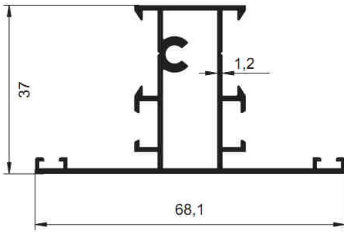
2150 - 0.735 kg/m
