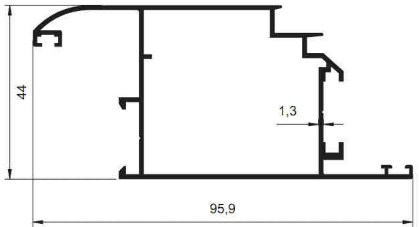
2160 - 0.971 kg/m
