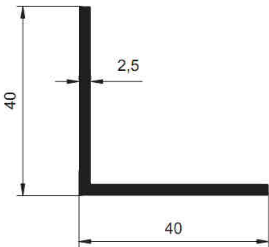
2204 - 0.523 kg/m
