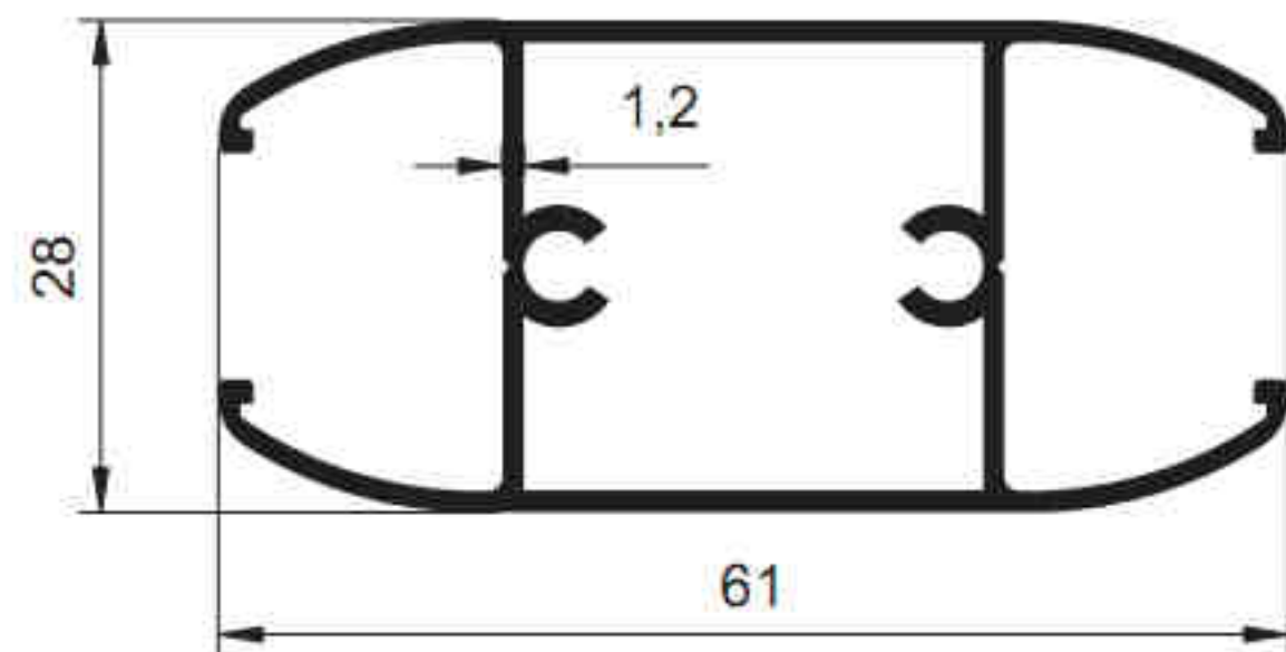
2171 - 0.700 kg/m
