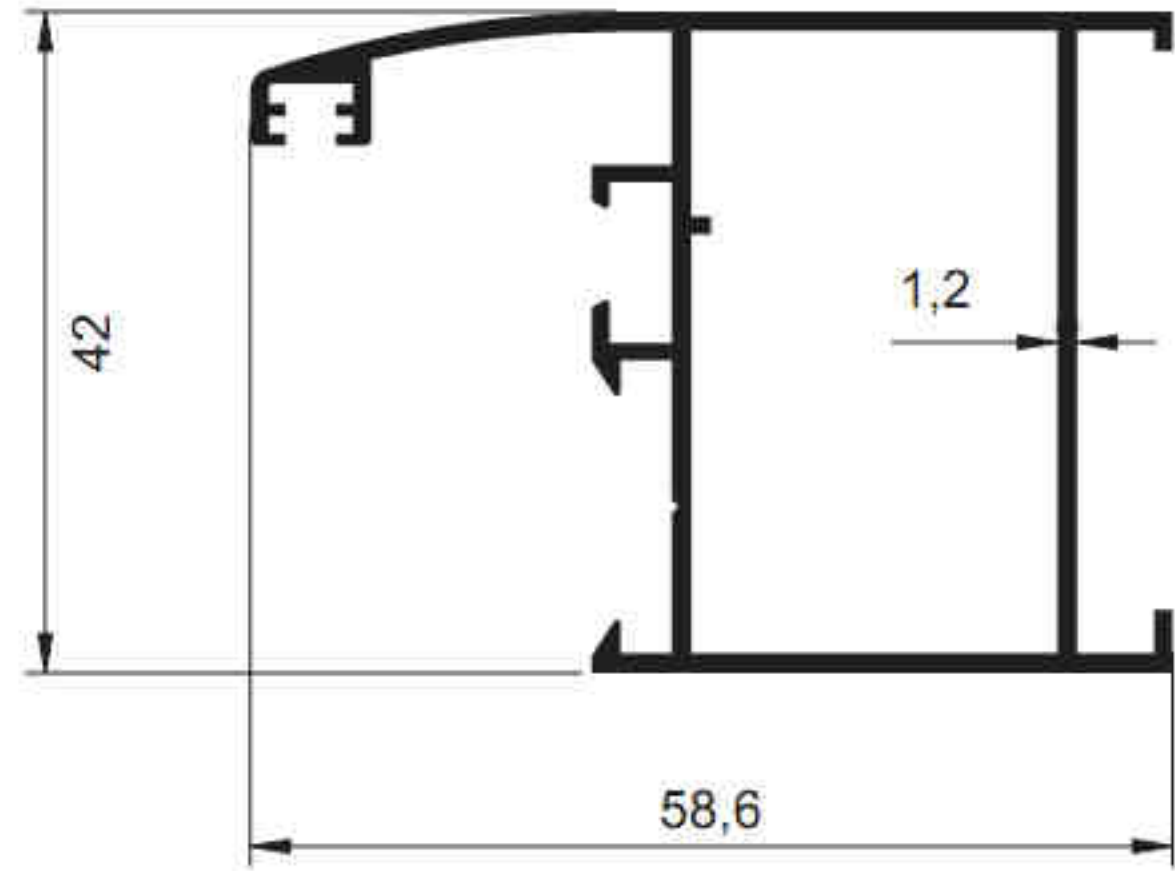
2163 - 0.705 kg/m
