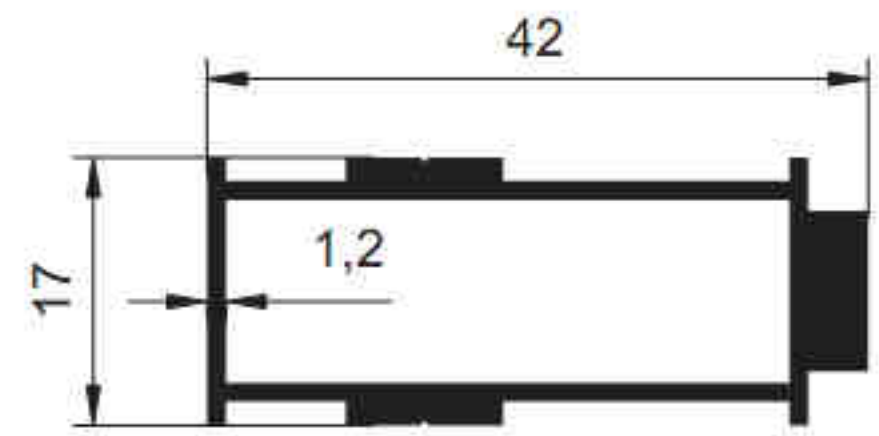
2250 - 0.527 kg/m
