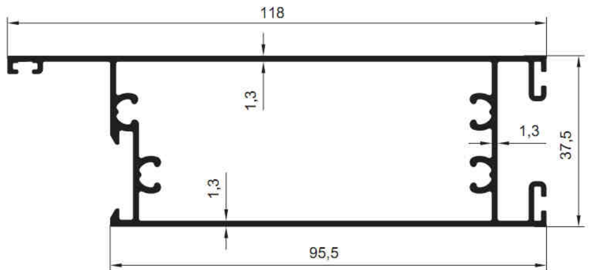
6008 - 1.338 kg/m
