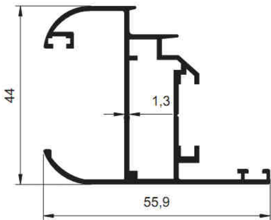
2222 - 0.749 kg/m
