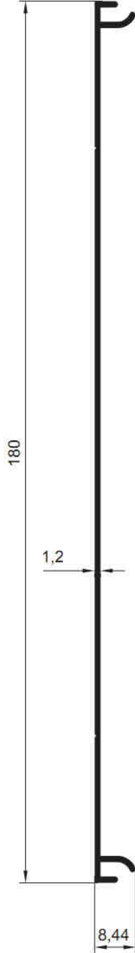
5581 - 0.663 kg/m
