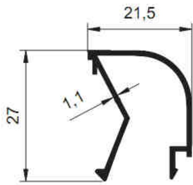
2152 - 0.246 kg/m
