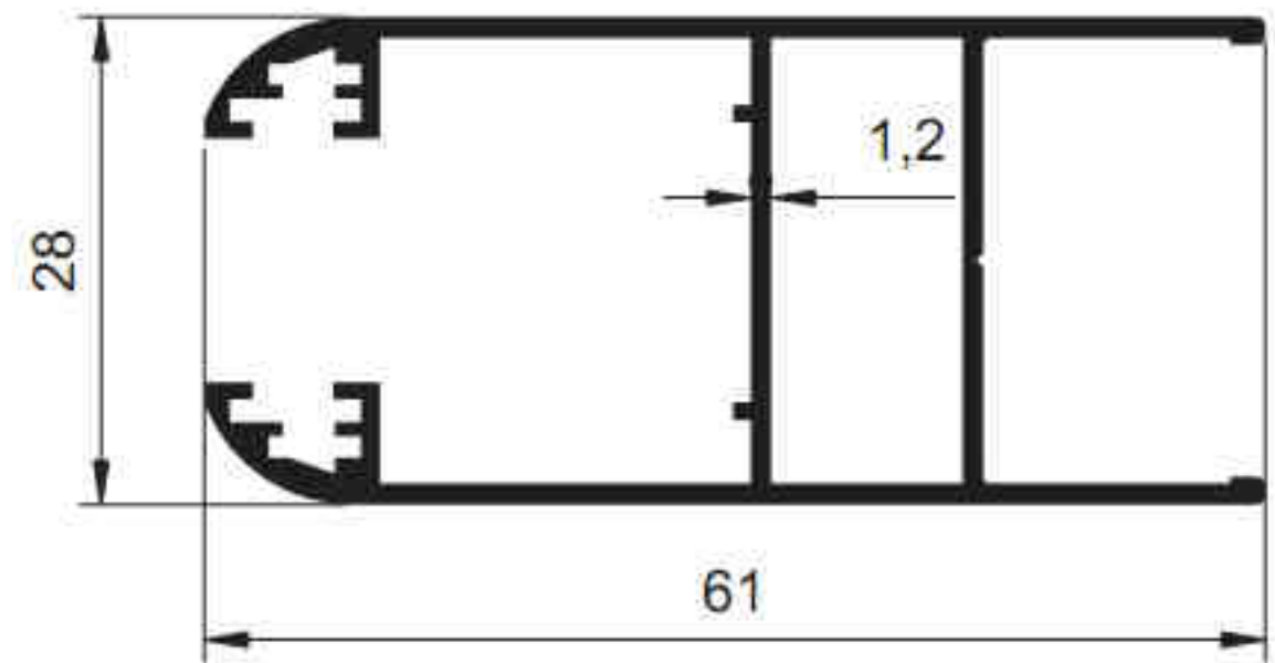
2157 - 0.682 kg/m
