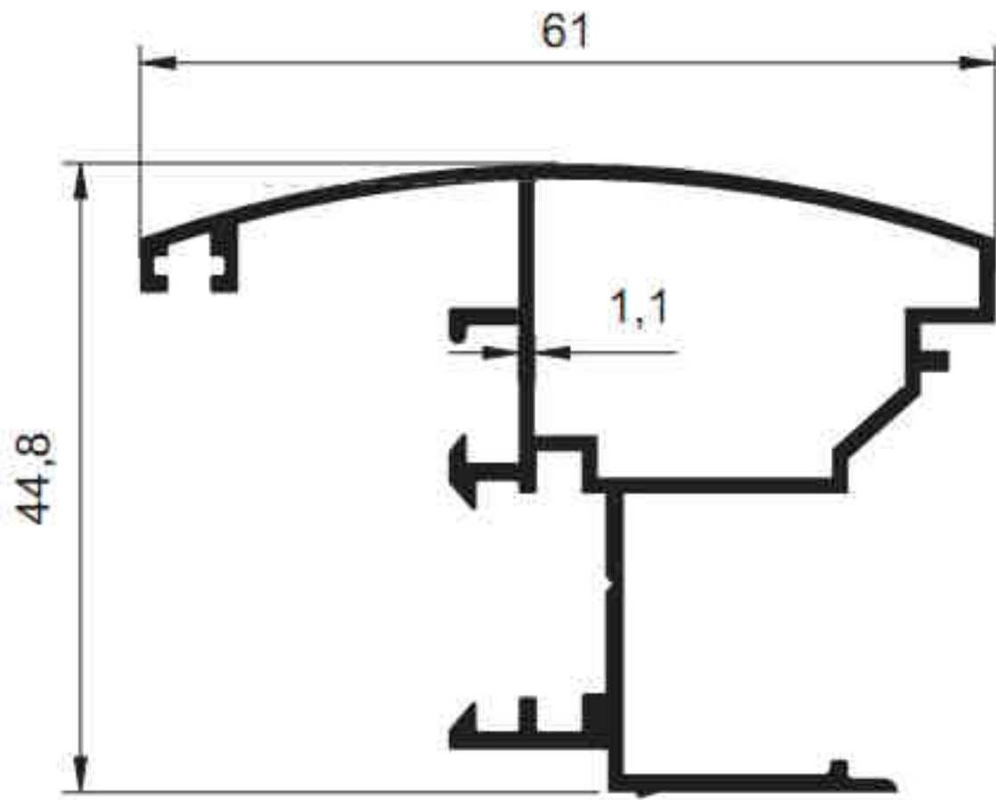
2159 - 0.722 kg/m
