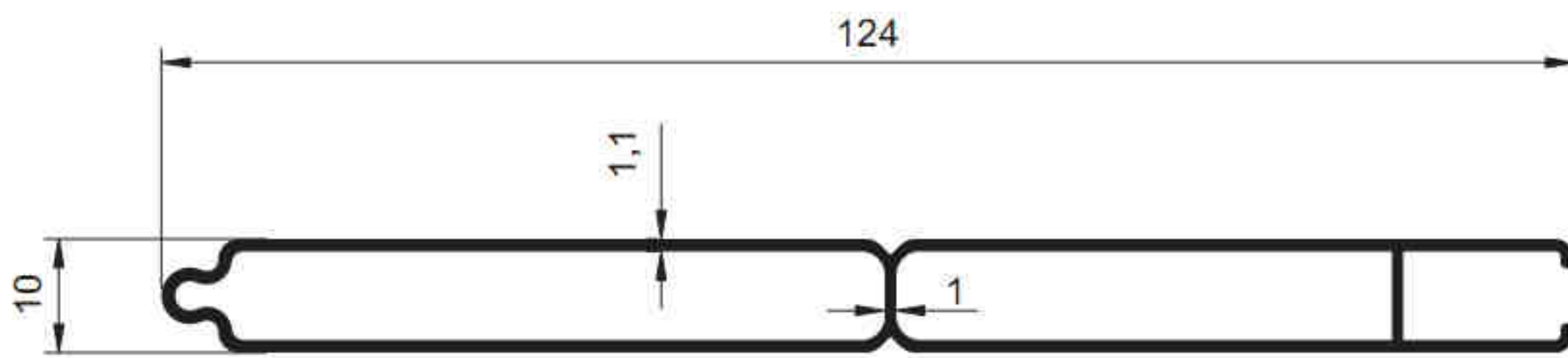
2154 - 0.802 kg/m
