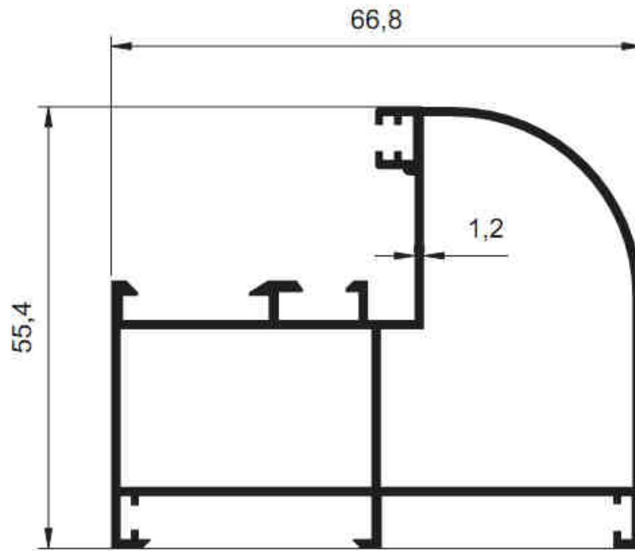
2161 - 1.002 kg/m
