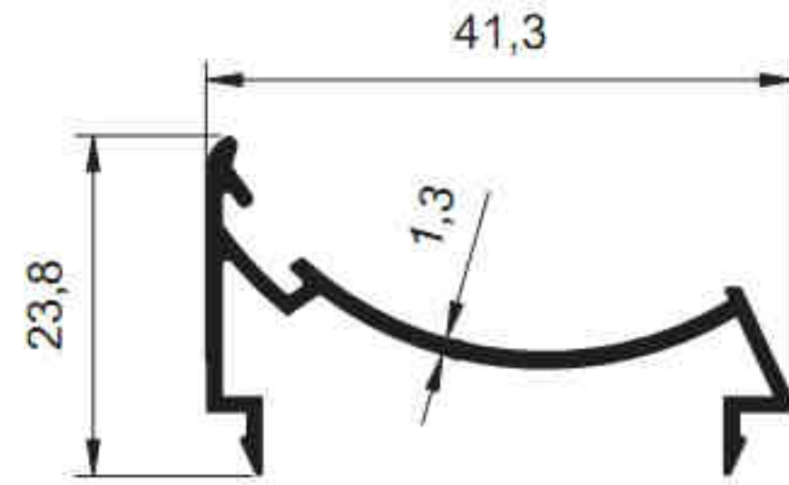
2220 - 0.299 kg/m
