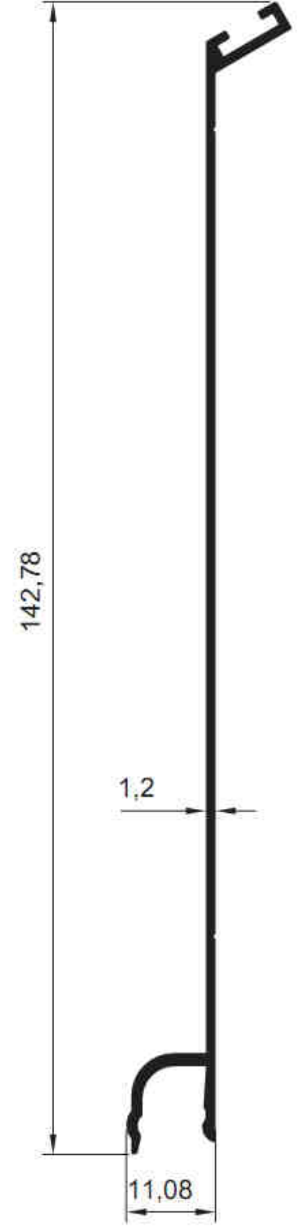
5583 - 0.581 kg/m
