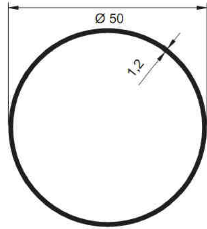
2221 - 0.497 kg/m
