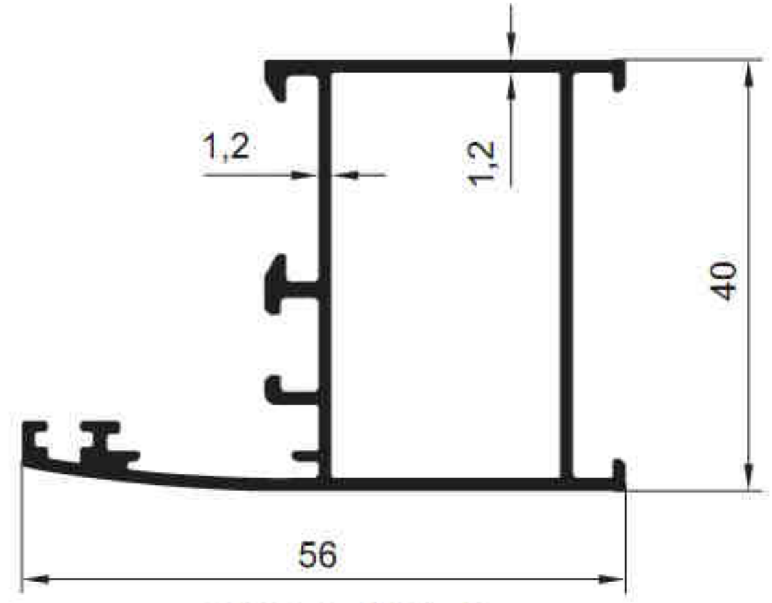
6004 - 0.681 kg/m
