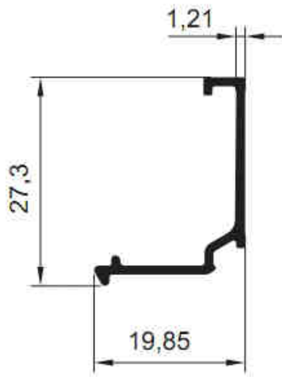
6007 - 0.176 kg/m
