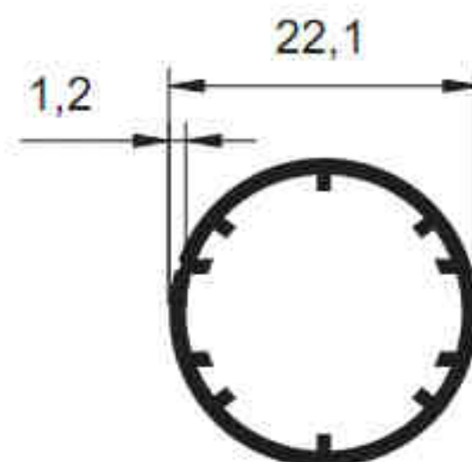
2218 - 0.246 kg/m
