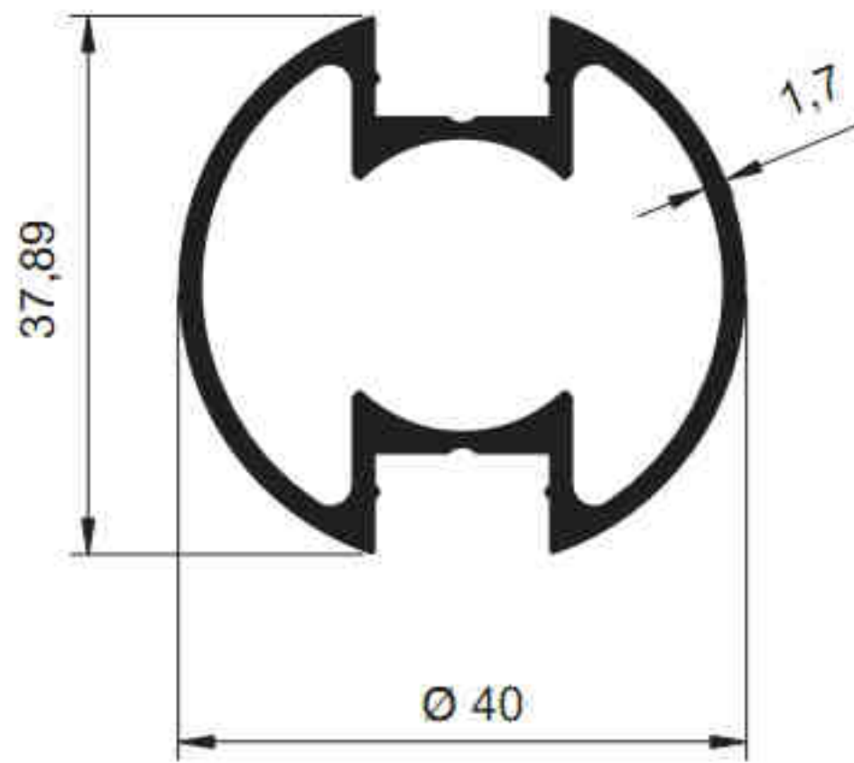
5075 - 0.775 kg/m
