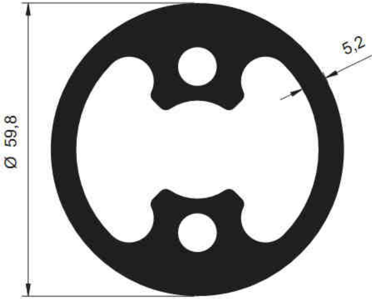
3888 - 3.837 kg/m
