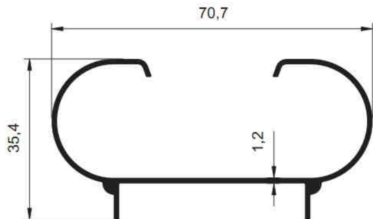
954 - 0.549 kg/m
