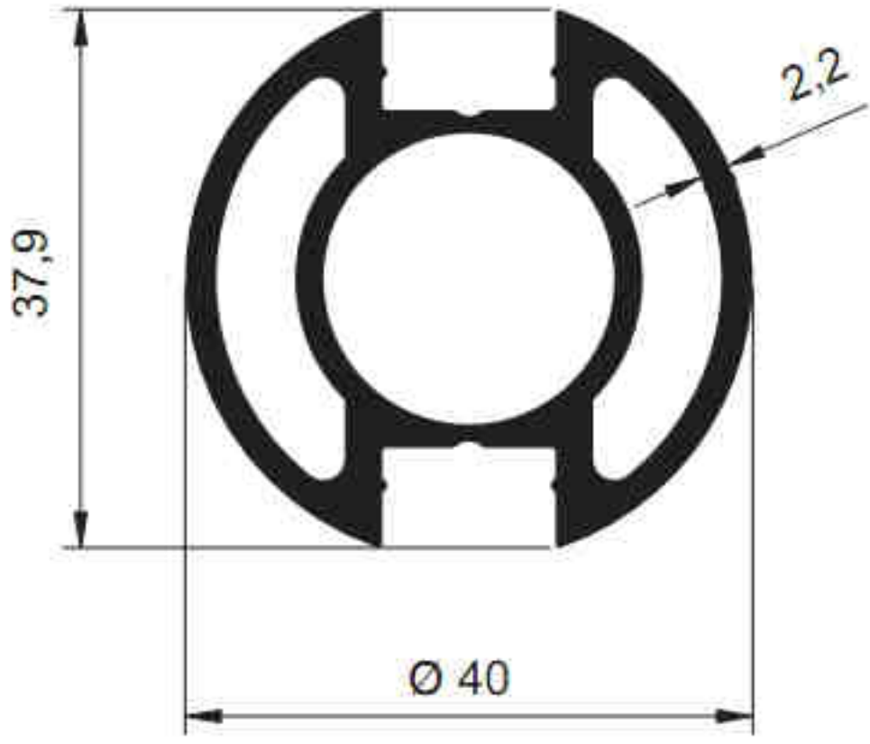
2207 - 1.156 kg/m
