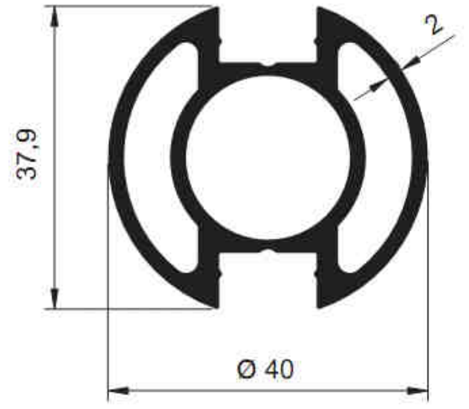
5082 - 1.115 kg/m
