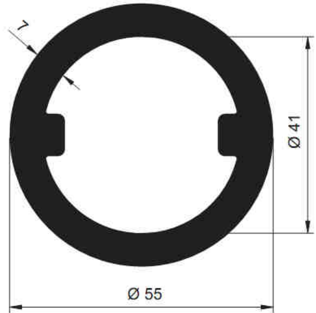
4347 - 3.056 kg/m
