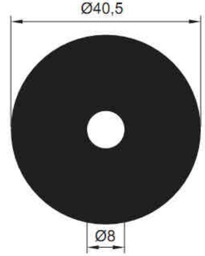
5246 - 3.343 kg/m
