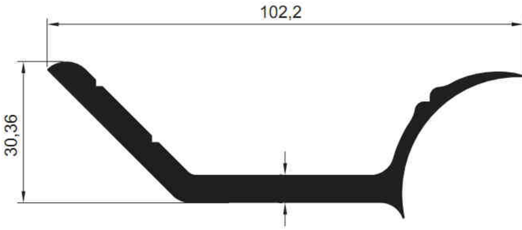
5568 - 1.661 kg/m
