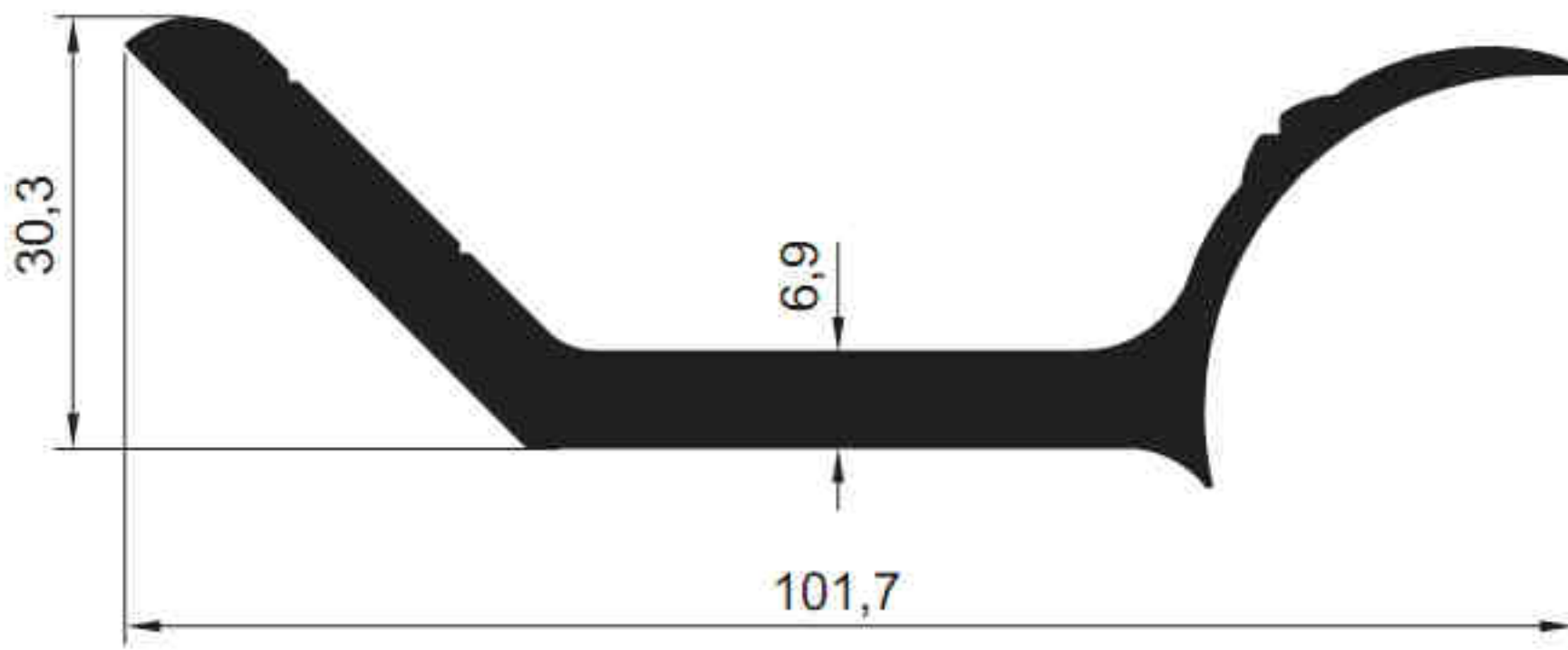
5253 - 1.869 kg/m
