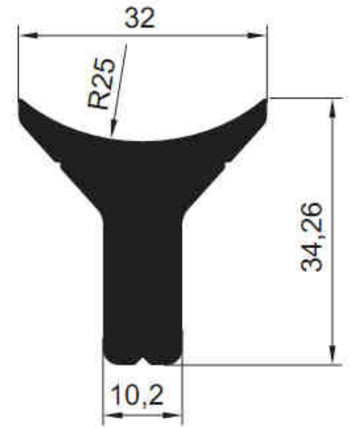
5184 - 1.150 kg/m
