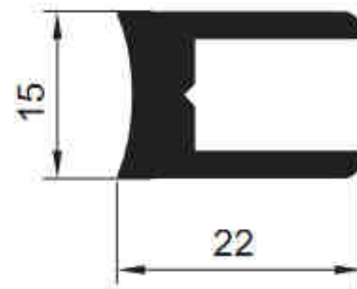
5557 - 0.446 kg/m
