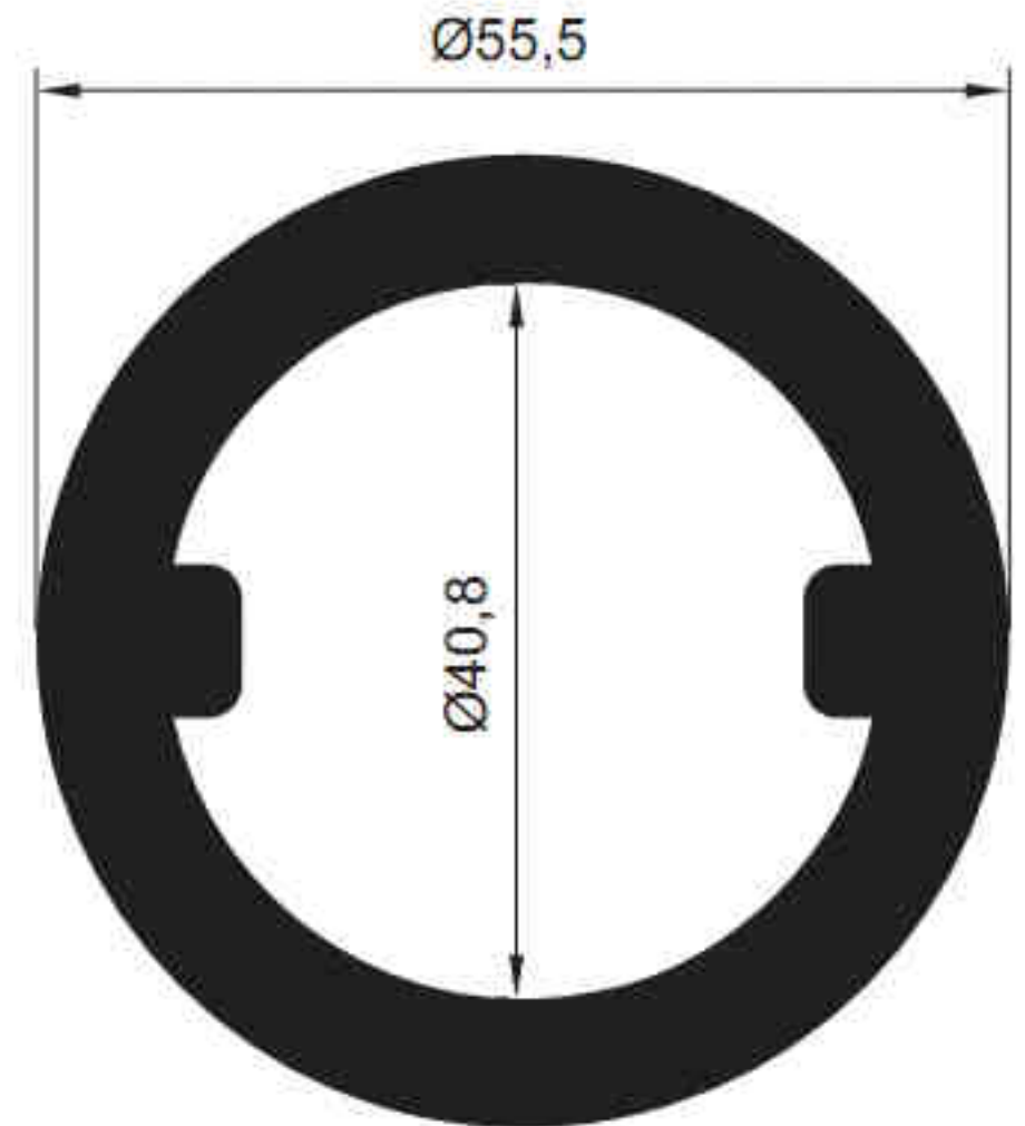
5457 - 3.194 kg/m
