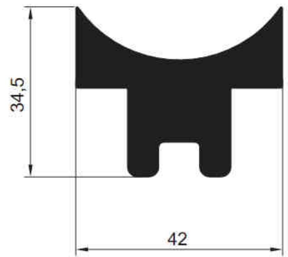
5549 - 1.890 kg/m
