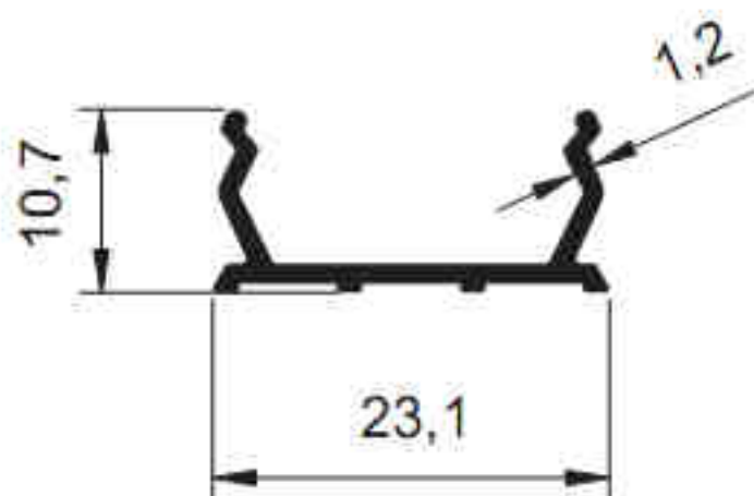
1048 - 0.147 kg/m
