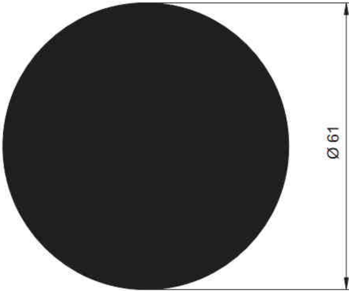
4508 - 7.889 kg/m
