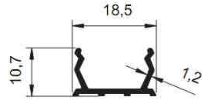
1053 - 0.129 kg/m
