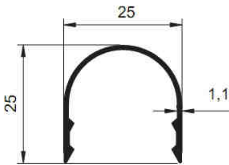
1047 - 0.208 kg/m
