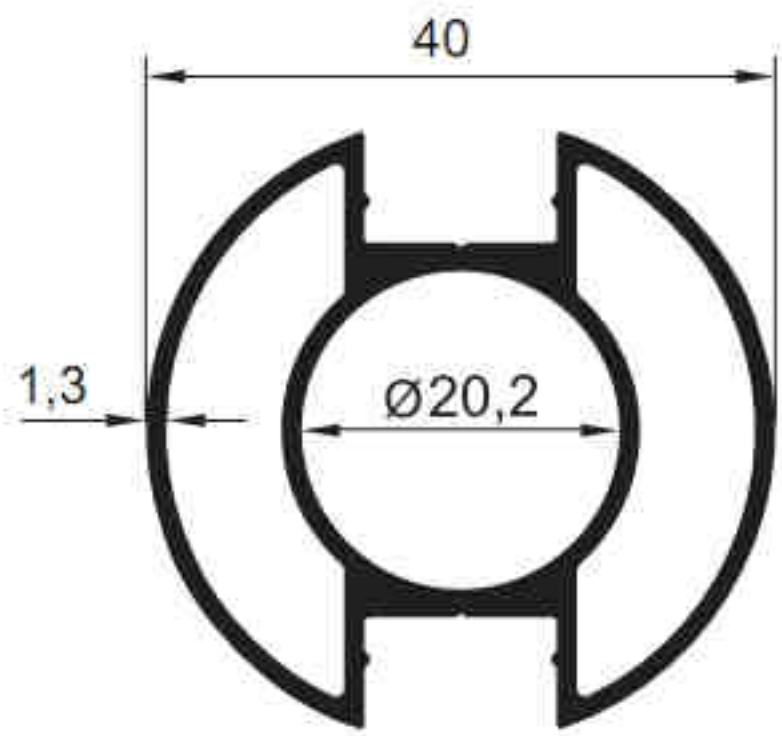
6393 - 0.770 kg/m
