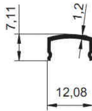
2208 - 0.065 kg/m
