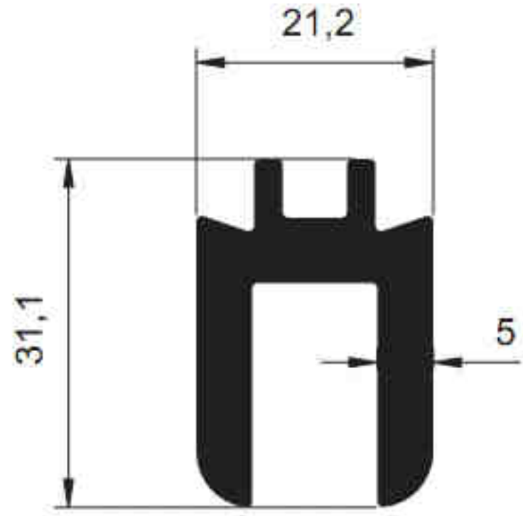
3887 - 0.904 kg/m
