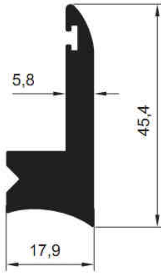
5249 - 1.002 kg/m
