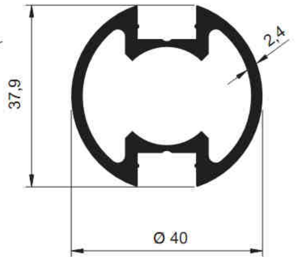
2518 - 1.005 kg/m
