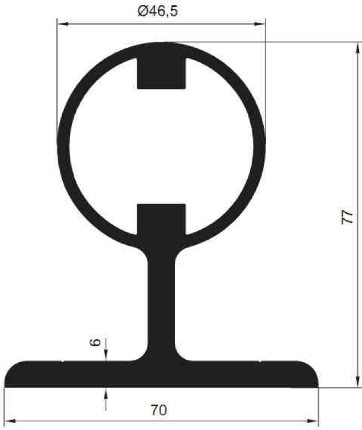
5251 - 2.995 kg/m
