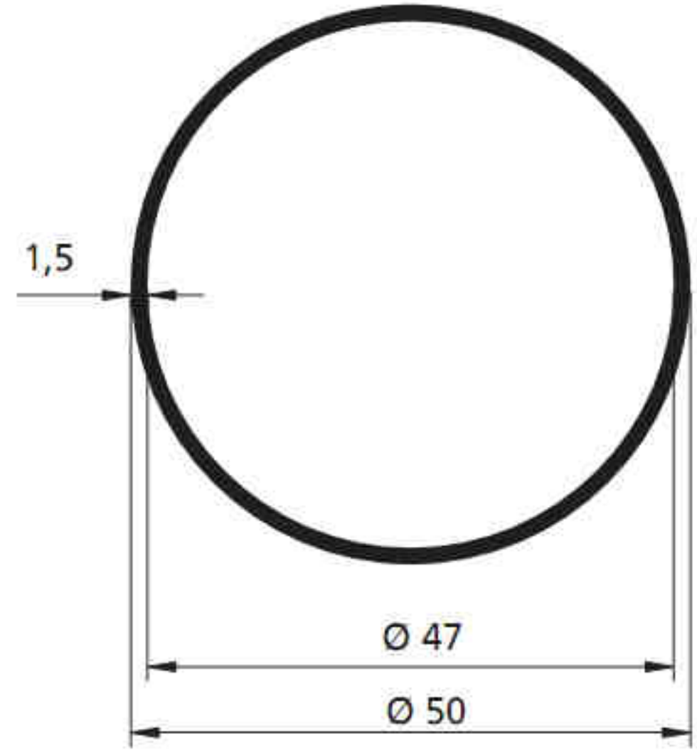
2395 - 0.617 kg/m
