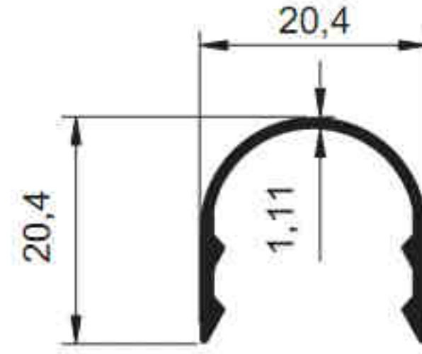
1052 - 0.180 kg/m
