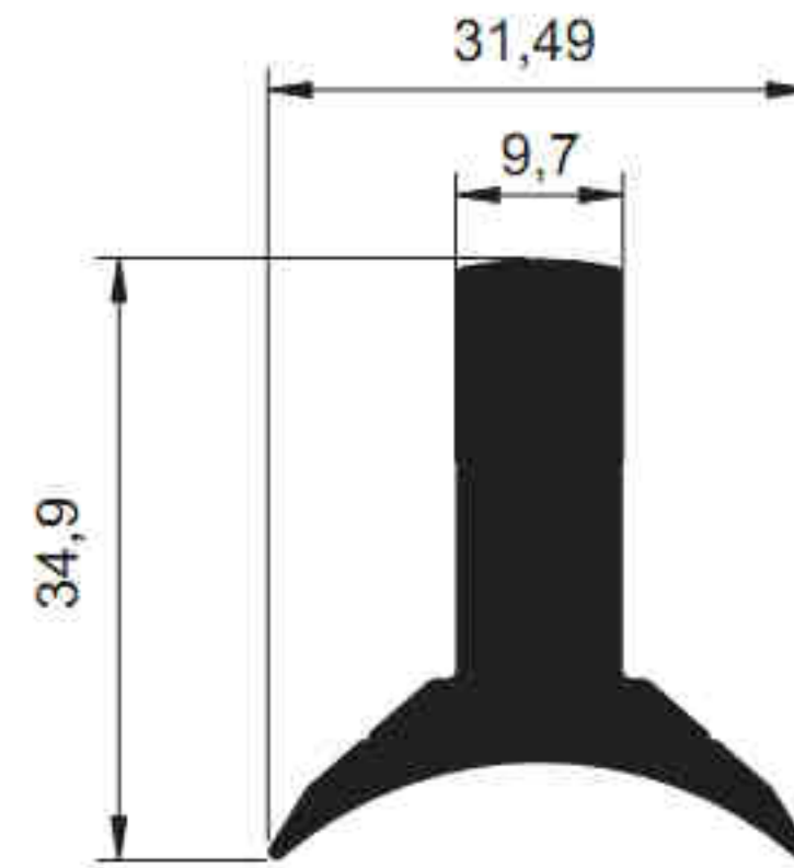
4513 - 0.993 kg/m
