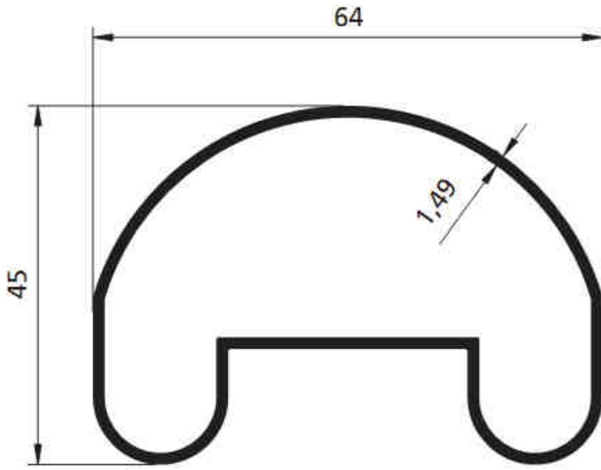
613 - 0.816 kg/m
