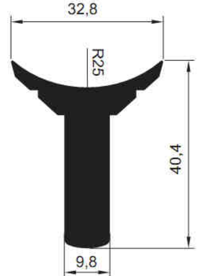
5248 - 1.192 kg/m
