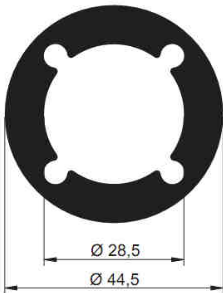
3369 - 2.263 kg/m
