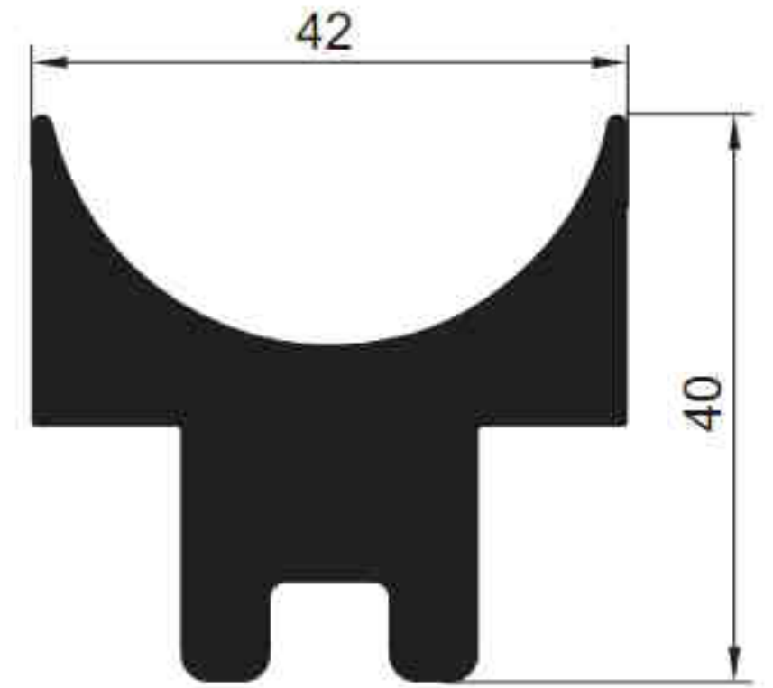
5562 - 2.059 kg/m
