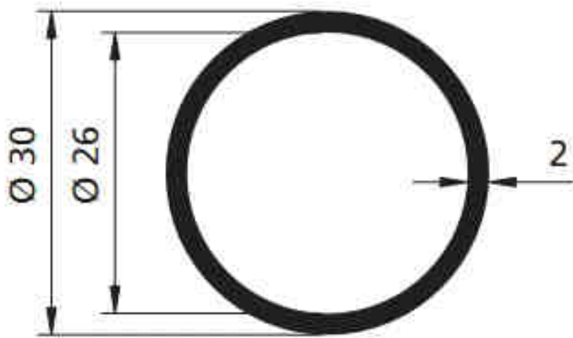
1095 - 0.475 kg/m
