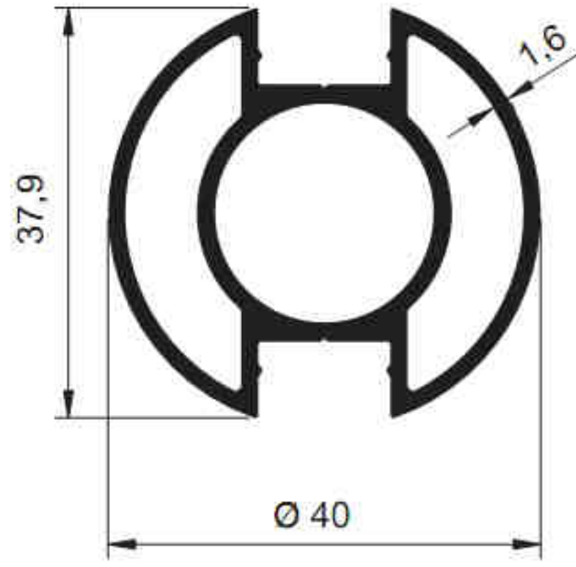
5035 - 0.906 kg/m
