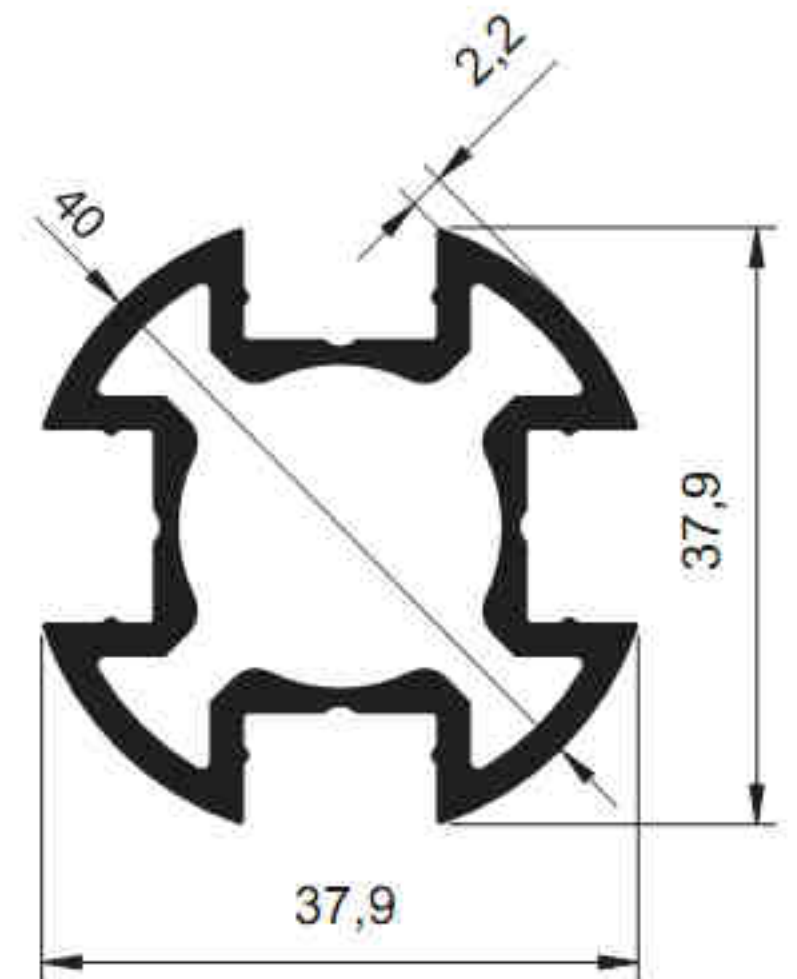
4658 - 0.999 kg/m
