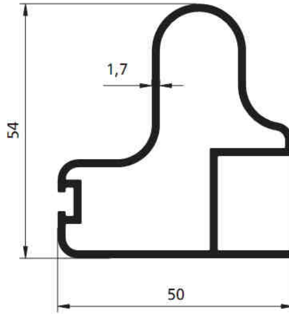
515 - 0.947 kg/m
