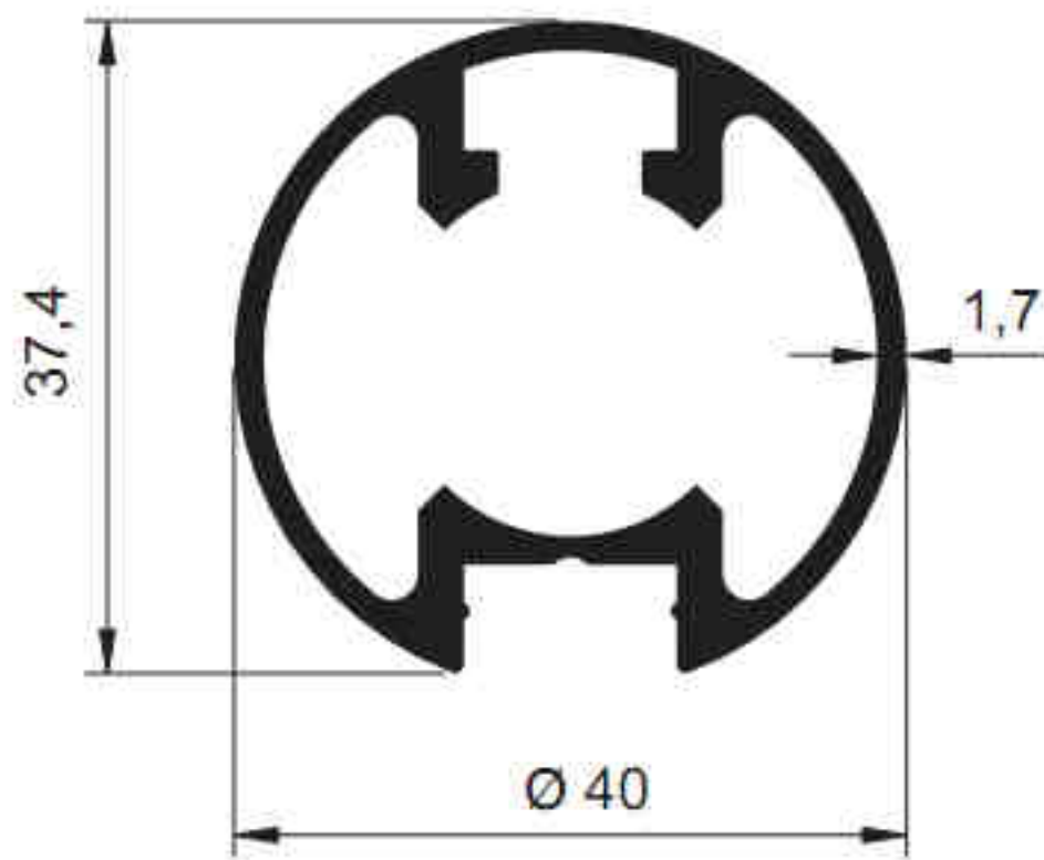
5046 - 0.833 kg/m
