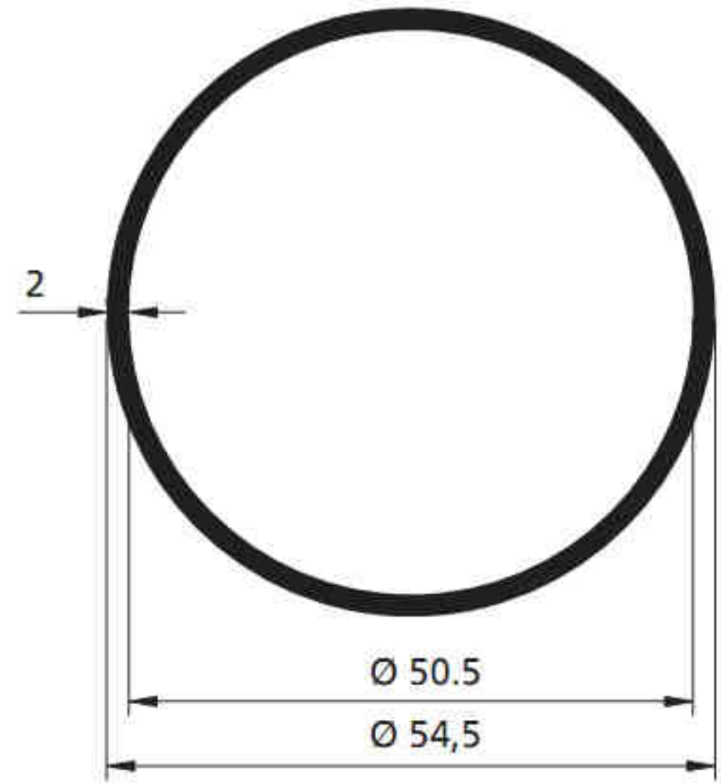
3884 - 0.890 kg/m
