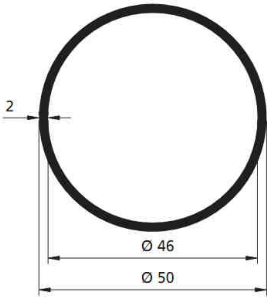
1129 - 1.814 kg/m
