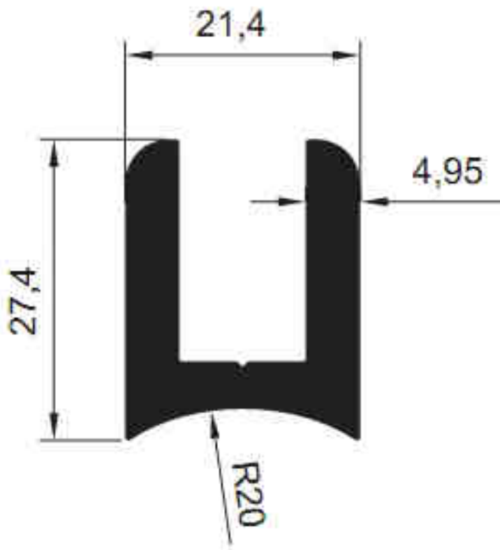
5243 - 0.829 kg/m
