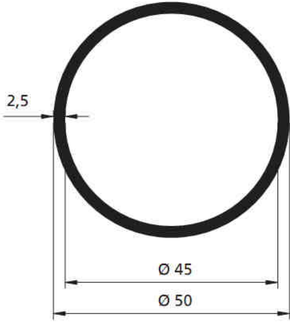
2517 - 1.007 kg/m
