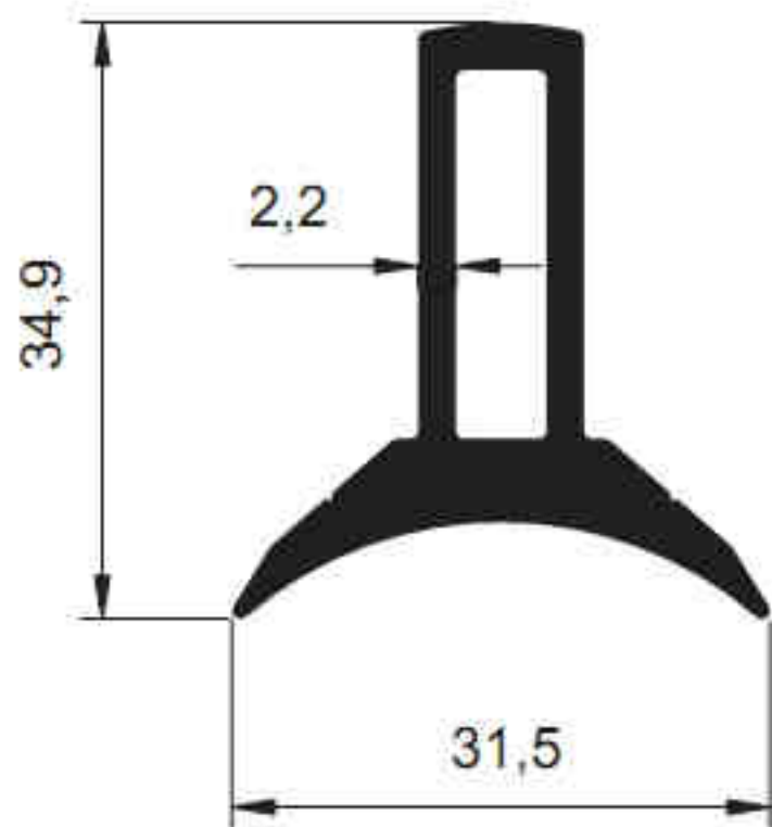
3882 - 0.685 kg/m
