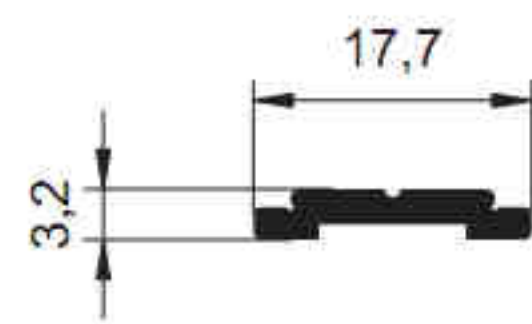
2790 - 0,111 Kg/m
