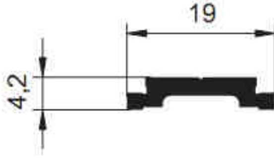
5254 - 0.138 kg/m
