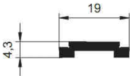
1523 - 0,149 Kg/m
