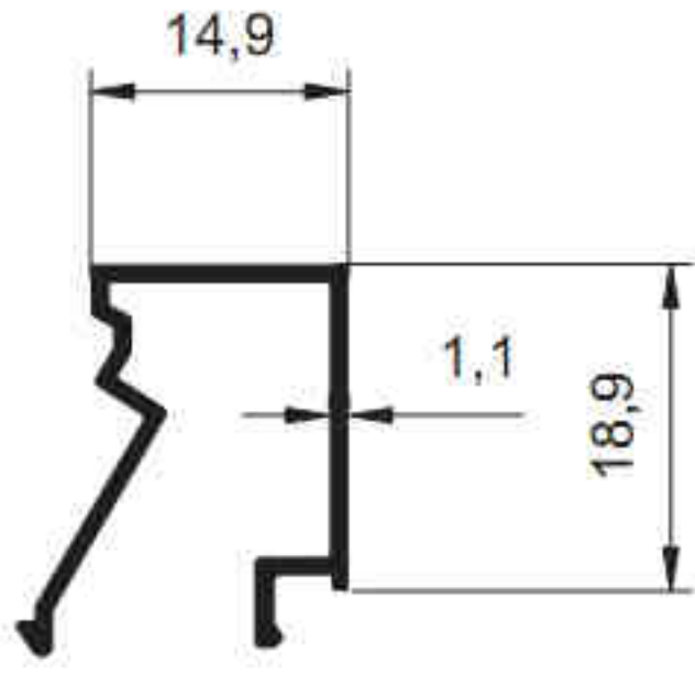
2506 - 0,205 Kg/m
