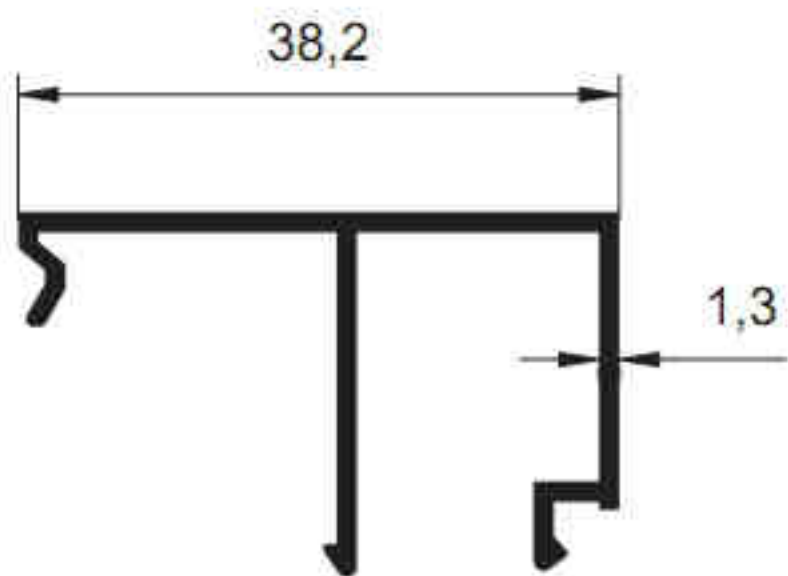
1507 - 0,330 Kg/m
