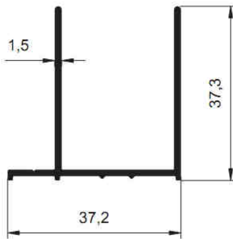
5220 - 0.435 kg/m
