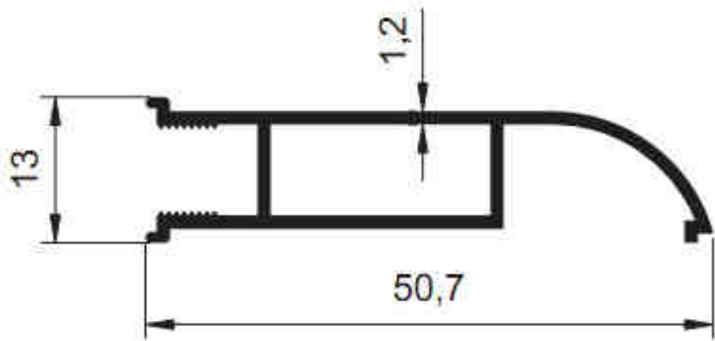
2016 - 0.353 kg/m
