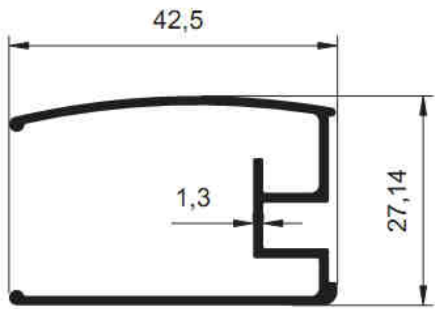
4598 - 0.444 kg/m
