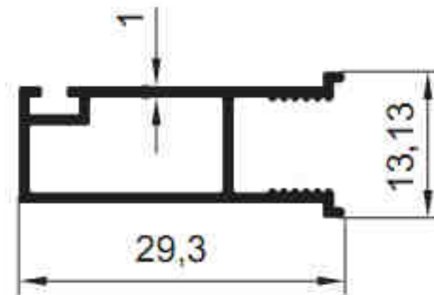
5693 - 0.232 kg/m
