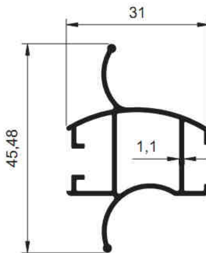
4600 - 0.424 kg/m
