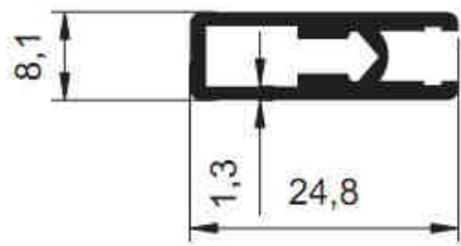
1968 - 0.266 kg/m
