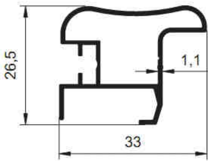
3038 - 0.360 kg/m
