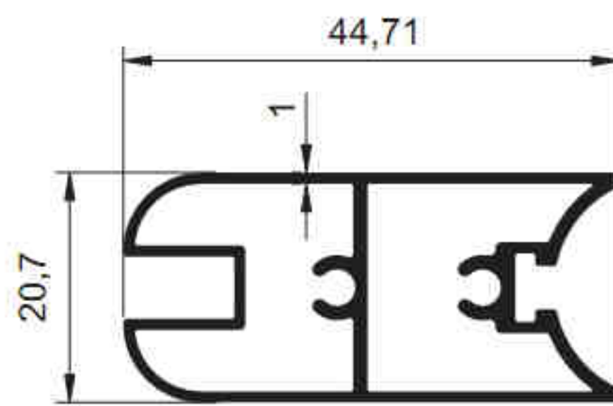
3337 - 0.574 kg/m
