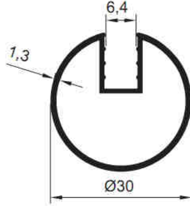
5384 - 0.384 kg/m
