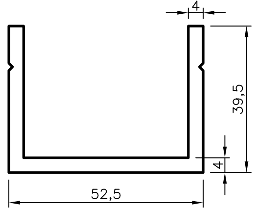
No : 3545 Kompozit Panel U Profili 1,350 kg/m
