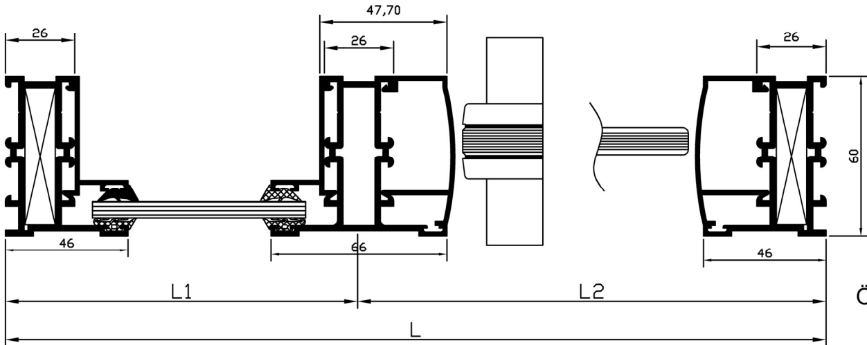
A-A Kesiti
